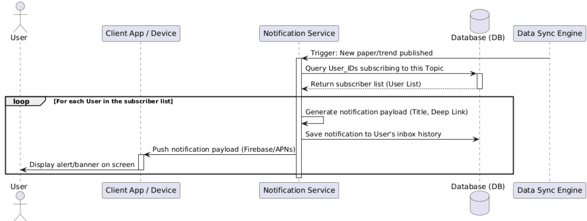
Hình 11: Sequence diagram
