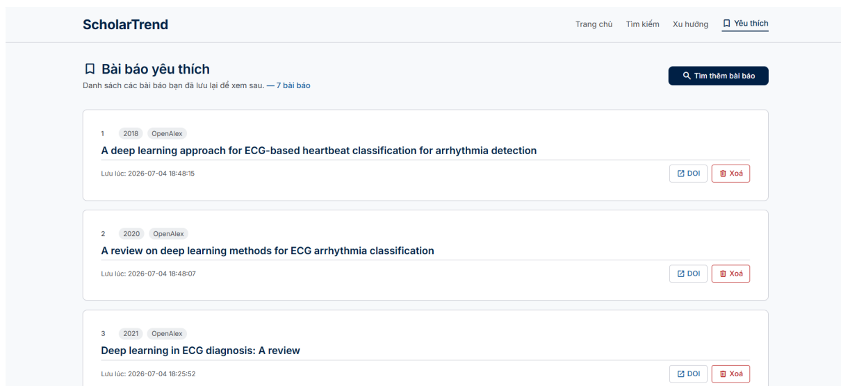
Hình 5: Bookmarked List
