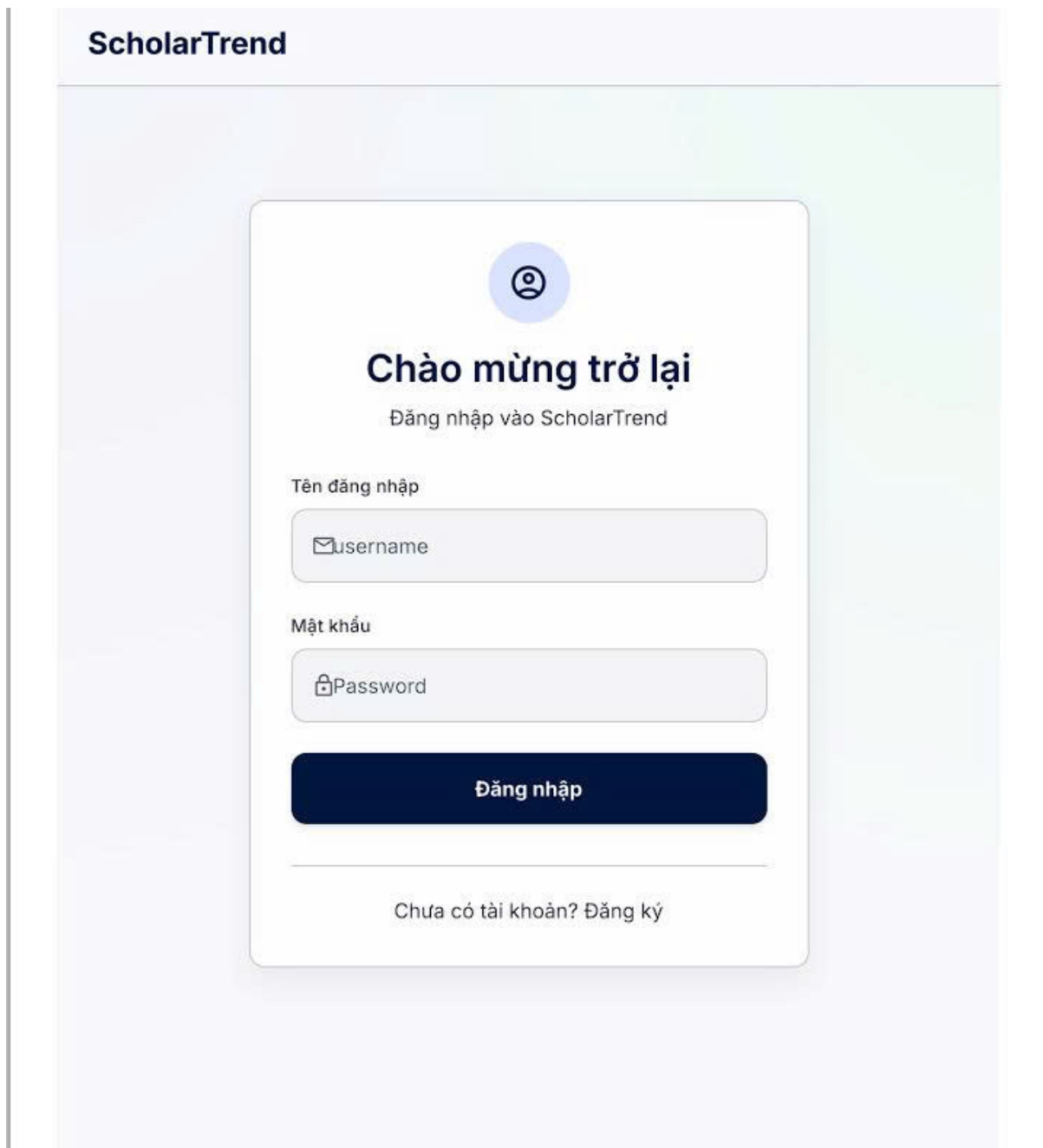
Hình 2: Login Page
