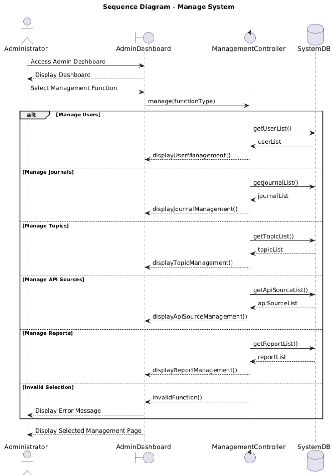
Hình 13: Sequence diagram
