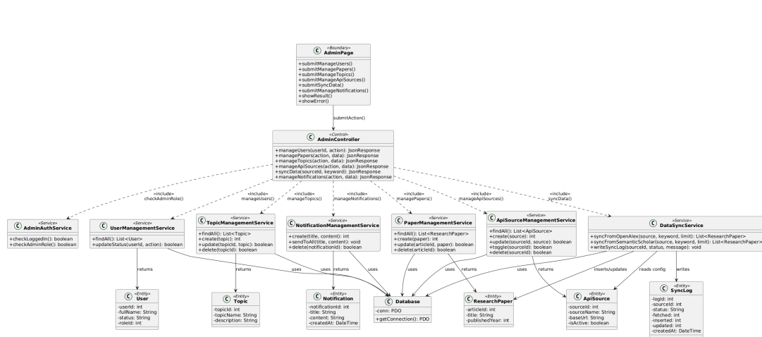
Hình 12: Class Diagram
