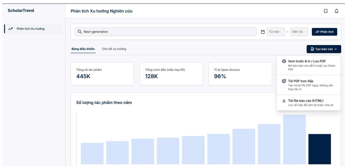
Hình 8: Generate Report
