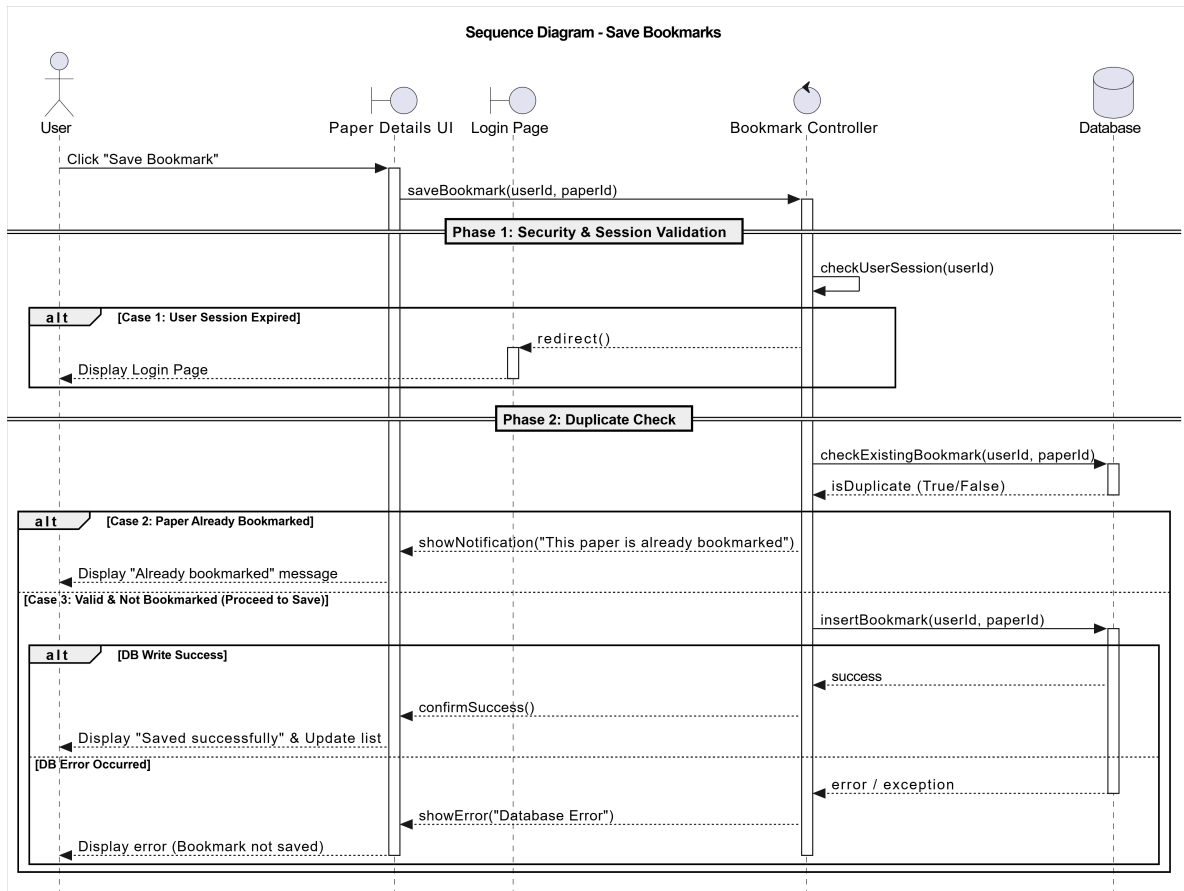
Hình 28: Sequence Diagram: Save Bookmarks
