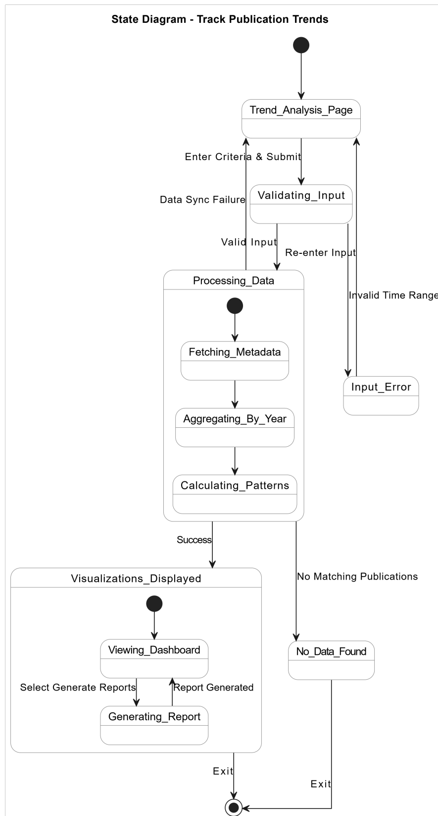
Hình 33: State Diagram: Track Publication Trends
