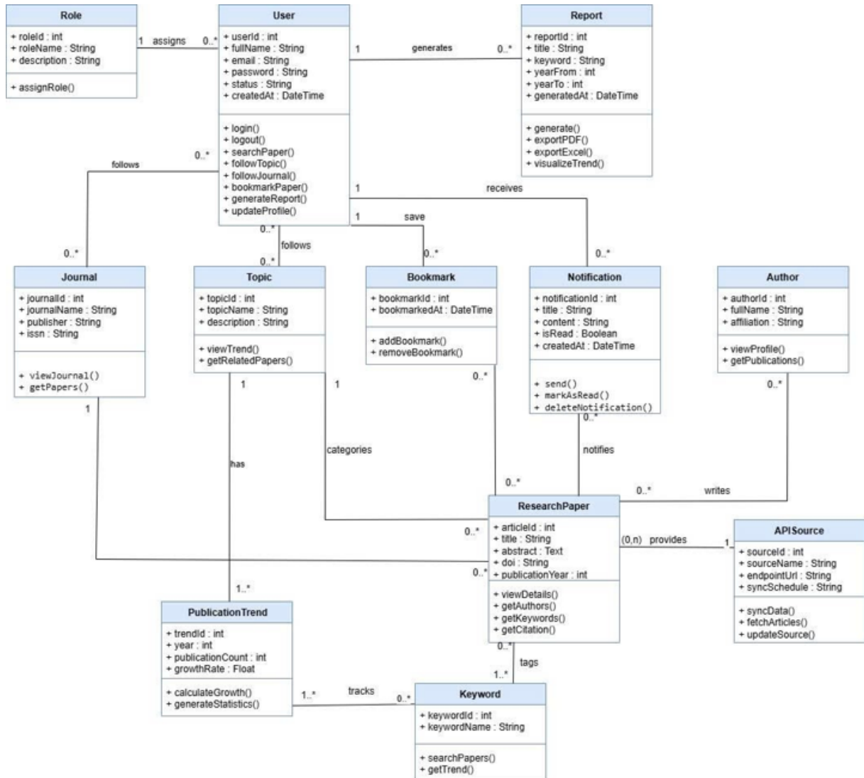
Hình 2: Class Diagram
