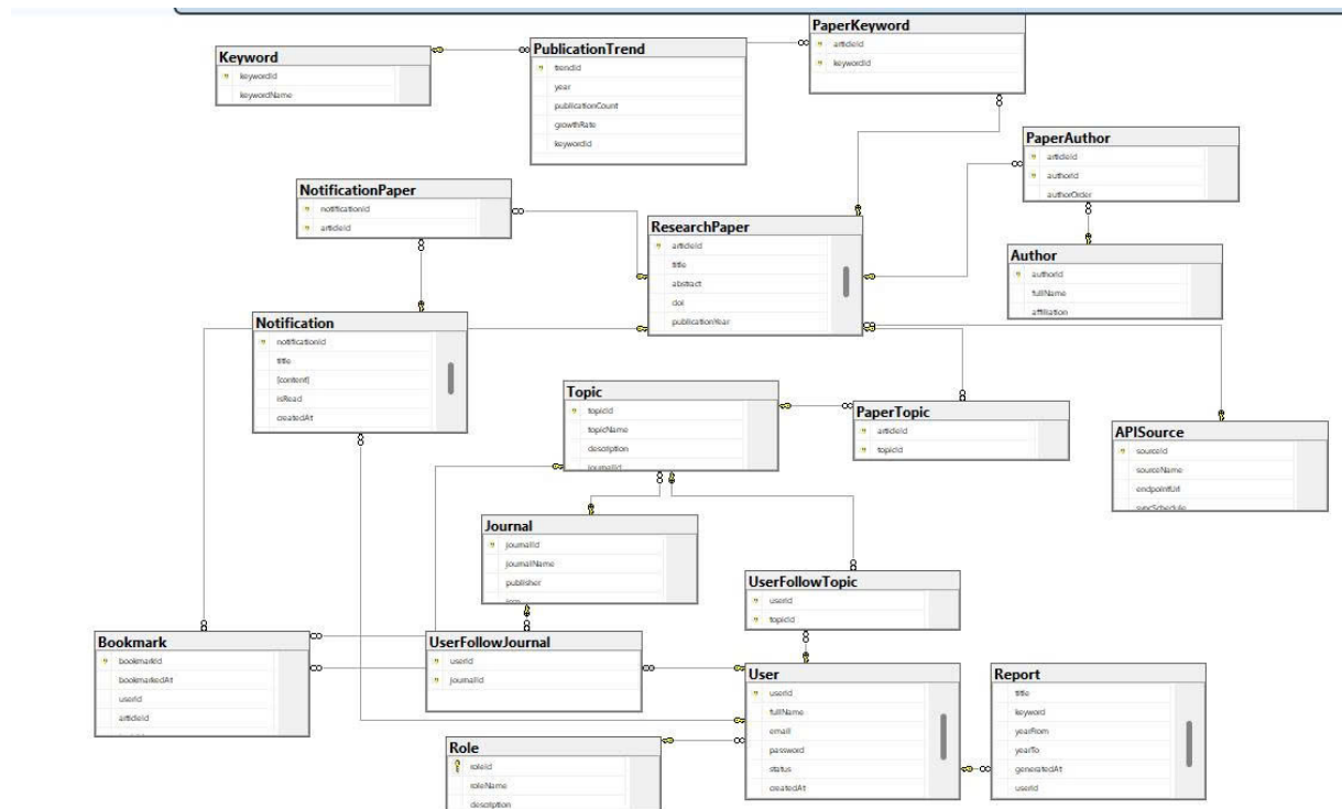
Hình 3: Database Design
