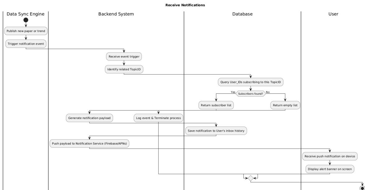
Hình 57: Activity diagram
