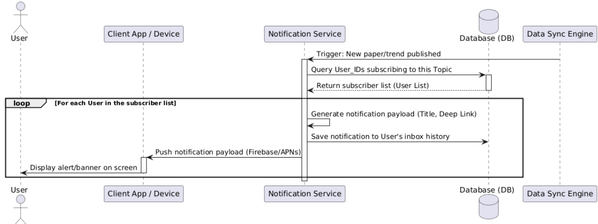
Hình 11: Sequence diagram
