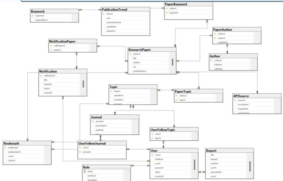
Hình 24: Database Design
