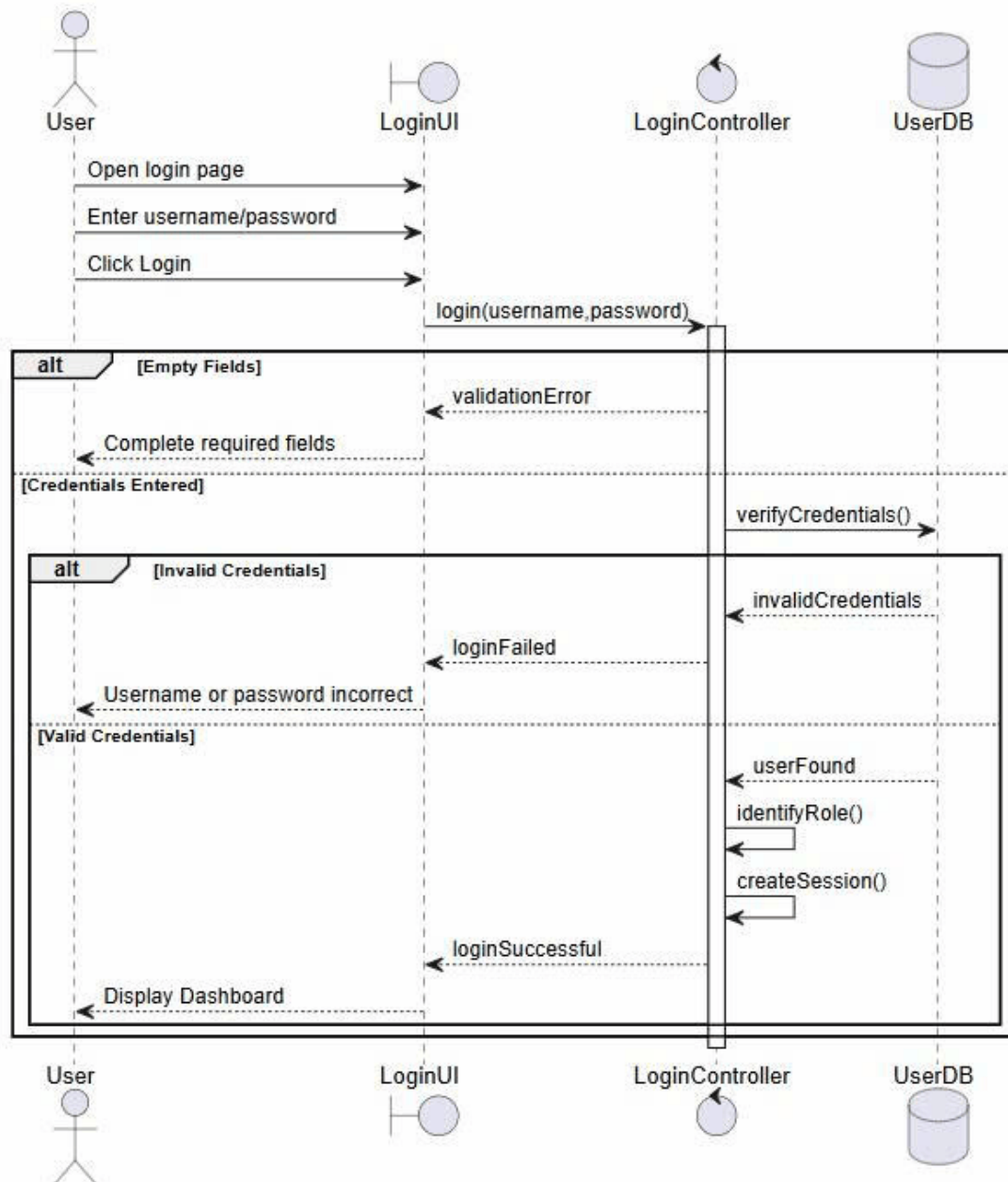
Hình 30: Sequence Diagram
