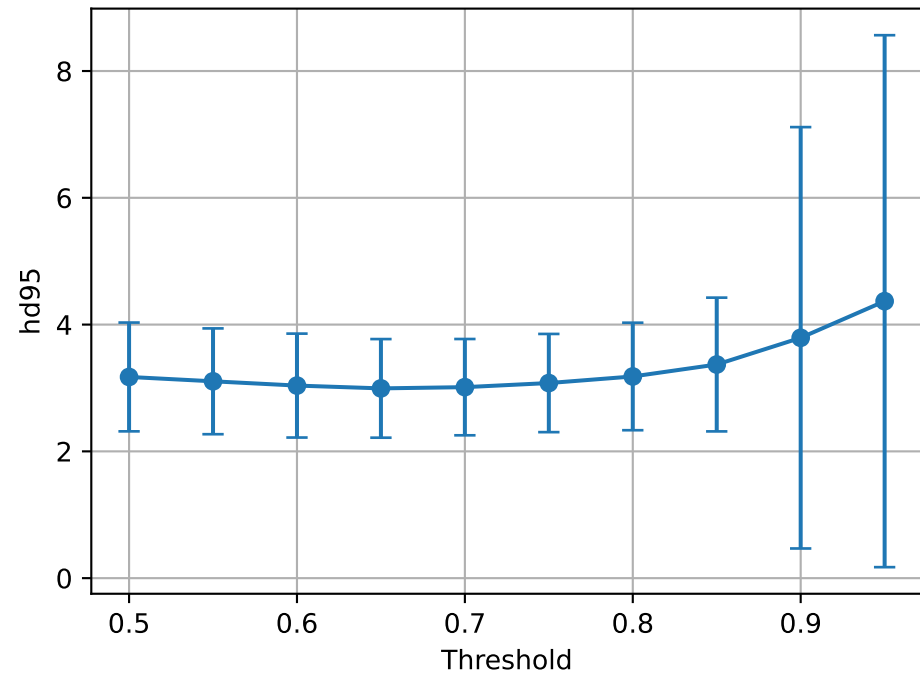
HD95
