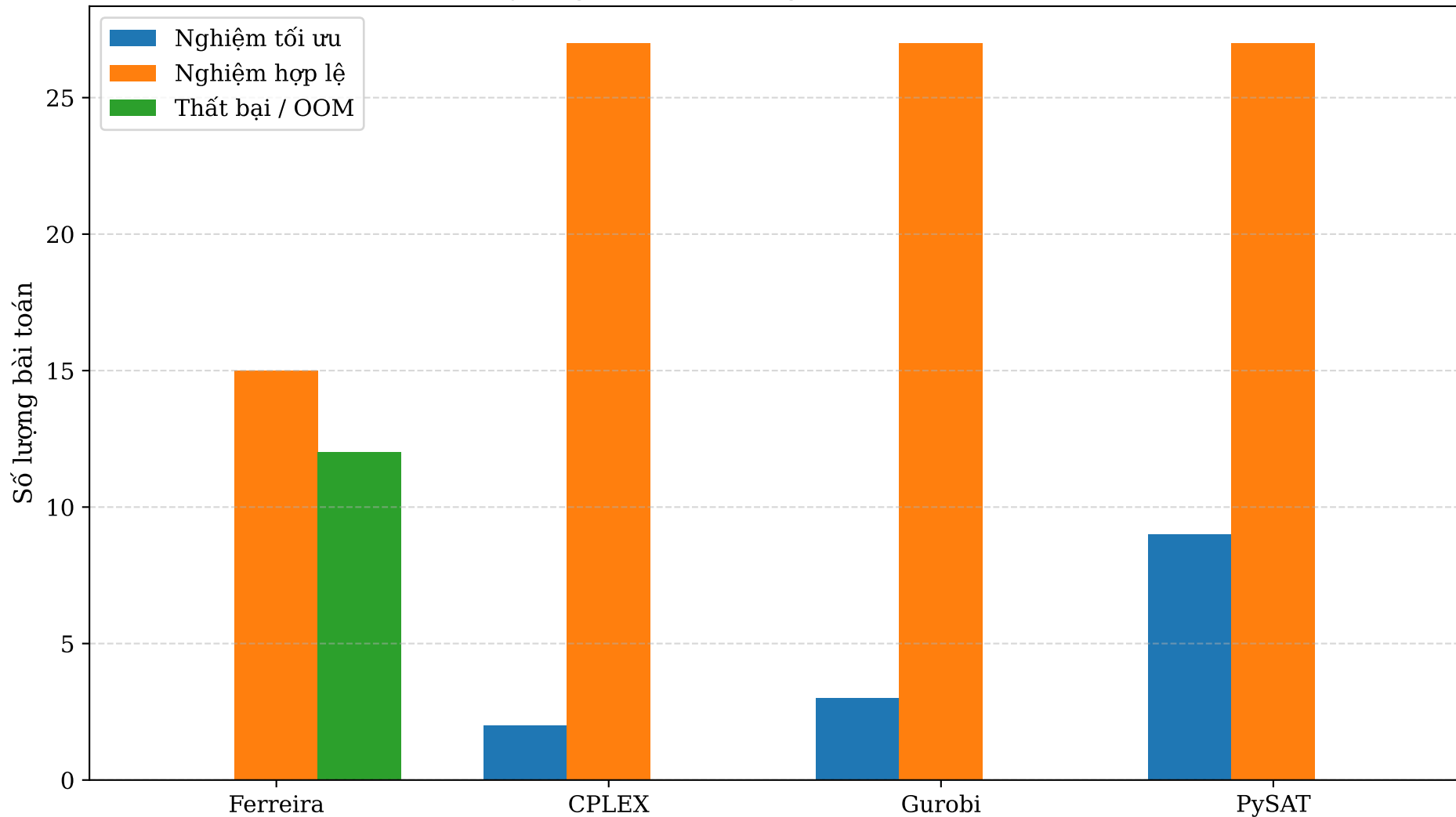
Tỷ lệ giải thành công trên bộ dữ liệu A
