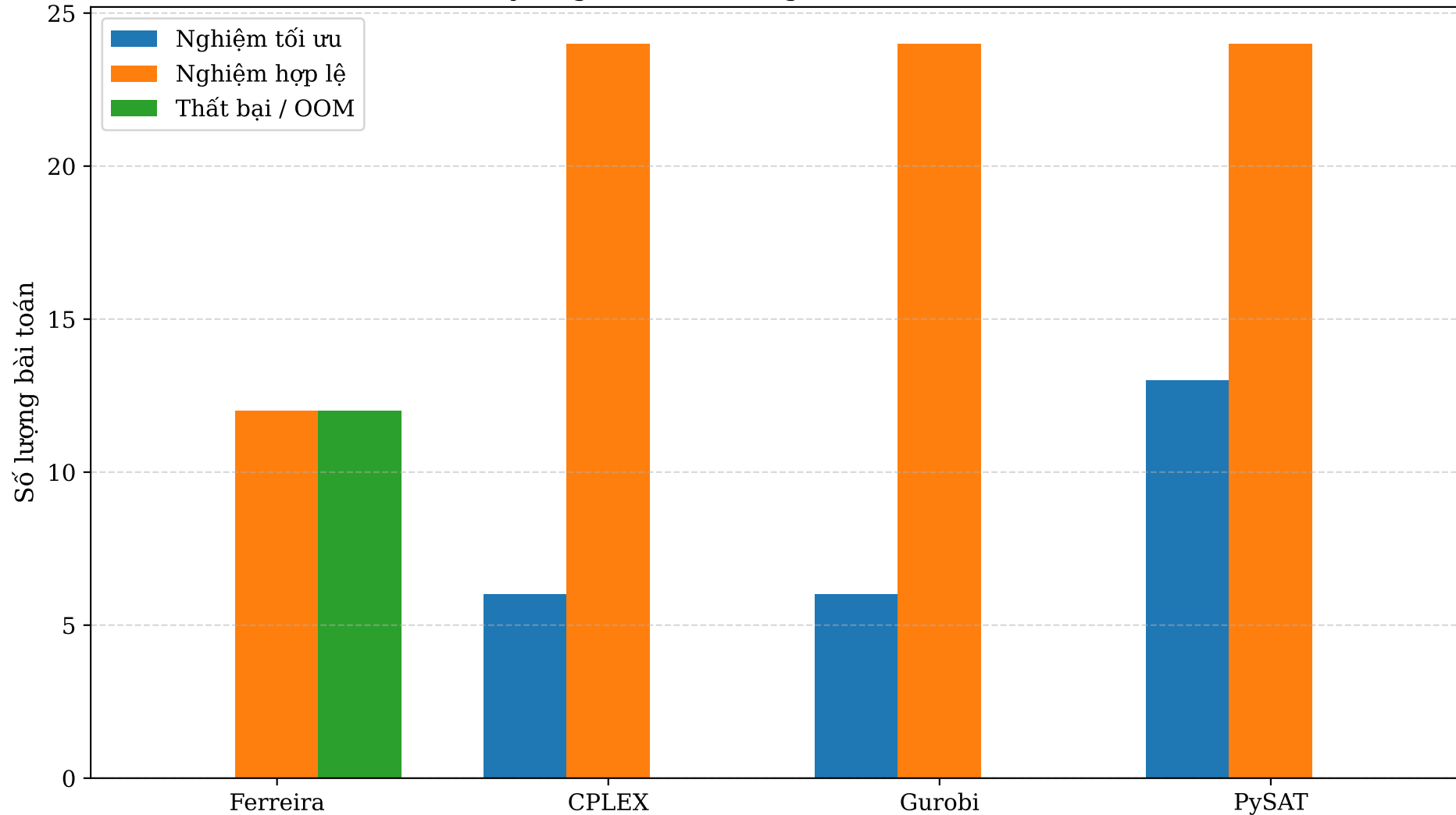
Tỷ lệ giải thành công trên bộ dữ liệu P
