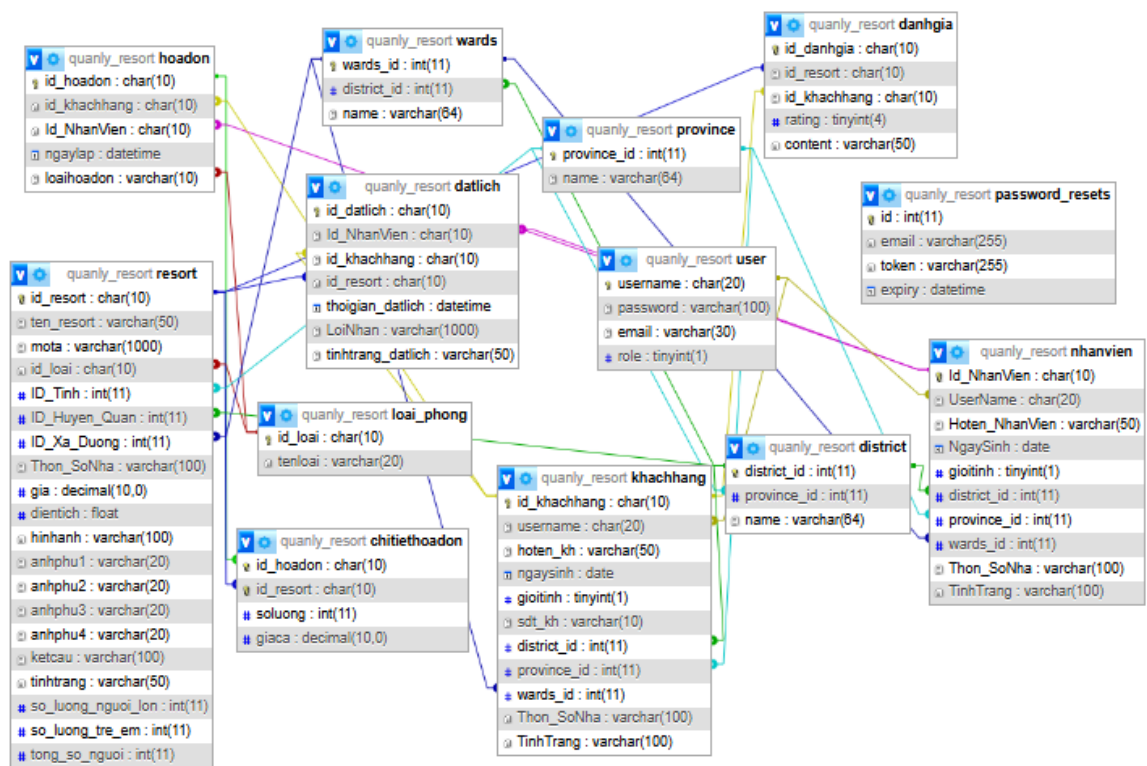
Hình 4.1: Sơ đồ ERD Diagram.
