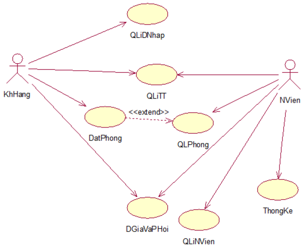
Hình 3.2: Sơ đồ Use-Case hệ thống.
