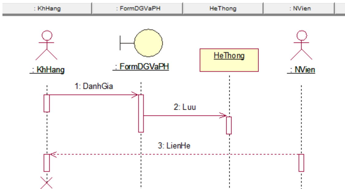
Hình 3.10: Sơ đồ tuần tự đánh giá và phản hồi.
