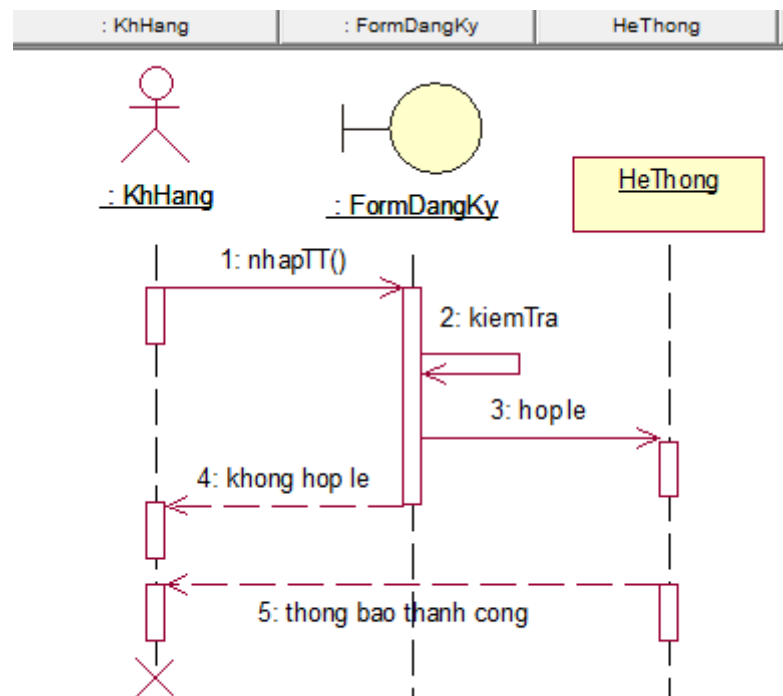
Hình 3.7: Sơ đồ tuần tự đăng kí.
