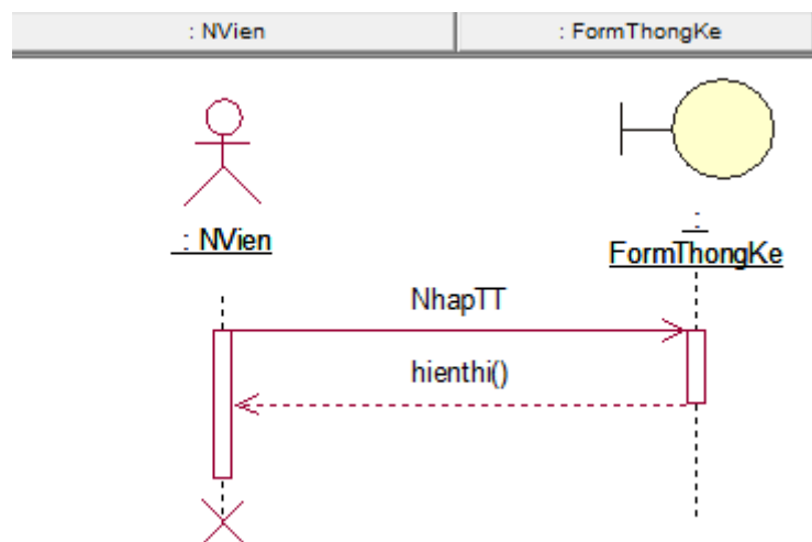
Hình 3.11: Sơ đồ tuần tự thống kê.
