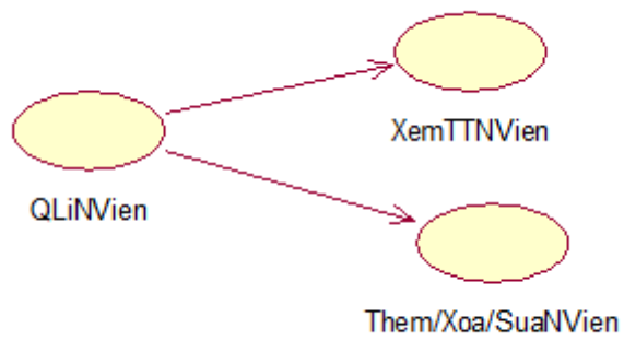
Hình 3.6: Sơ đồ Use-Case quản lí nhân viên.
