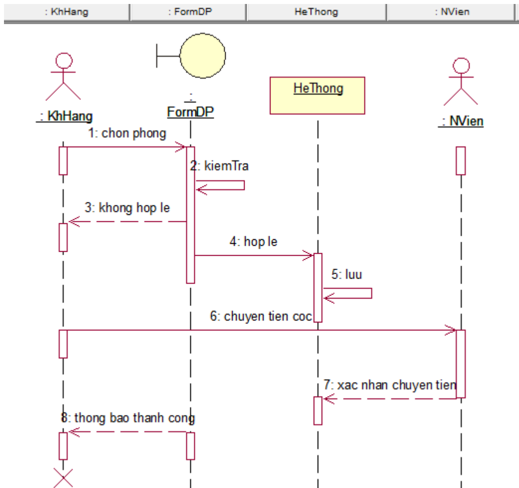
Hình 3.9: Sơ đồ tuần tự đặt phòng.
