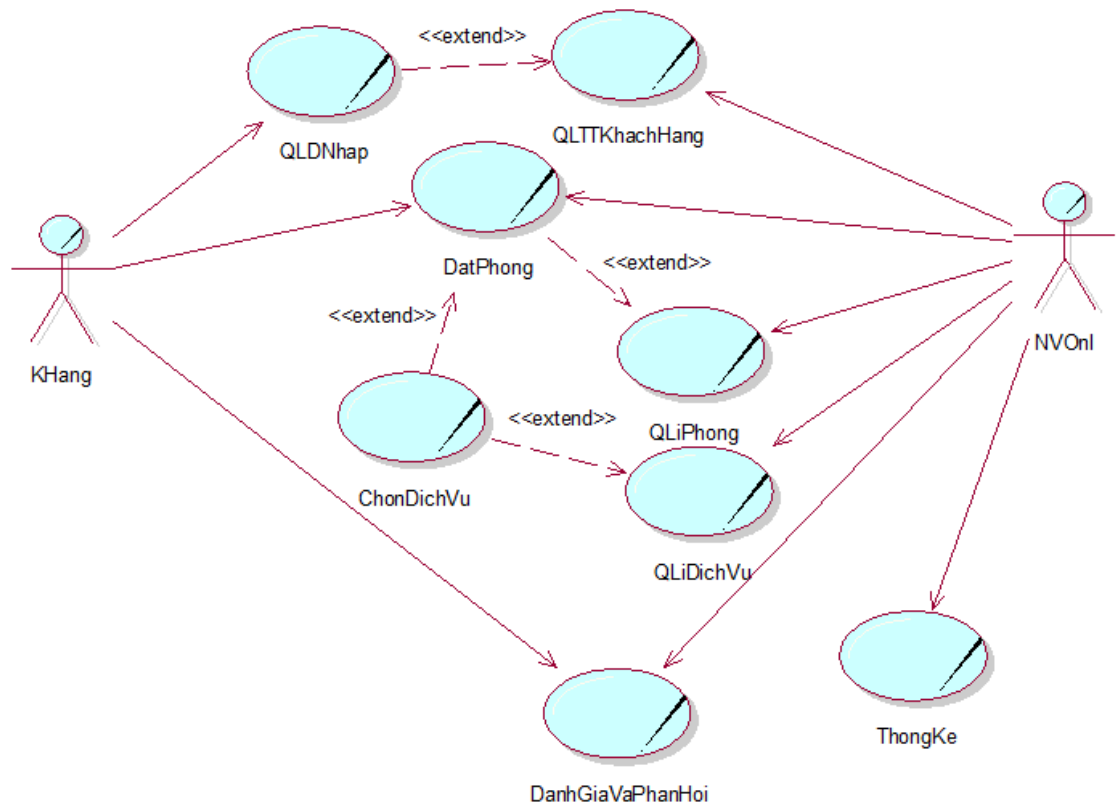
Hình 3.1: Sơ đồ use-case nghiệp vụ
