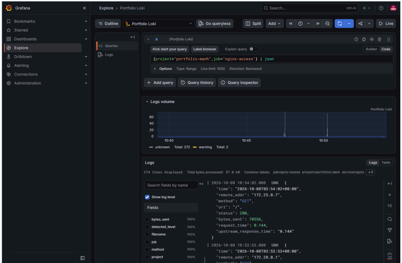
Hình 16. Grafana Explore / Portfolio Loki: truy vấn JSON access logs và dữ liệu thực.
