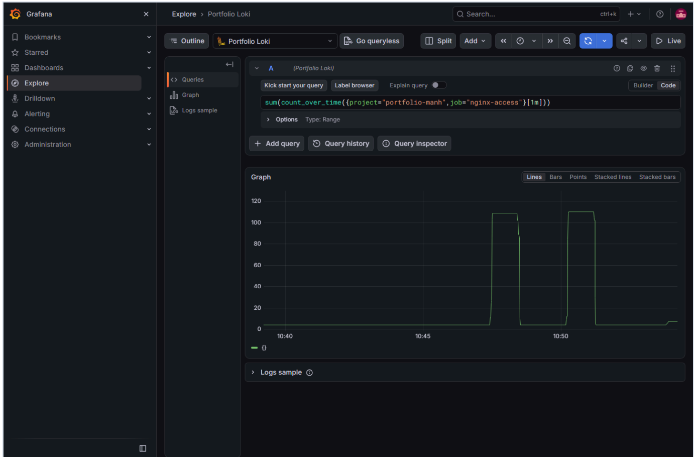
Hình 18. Grafana Explore: biểu đồ số request trong từng cửa sổ một phút.
