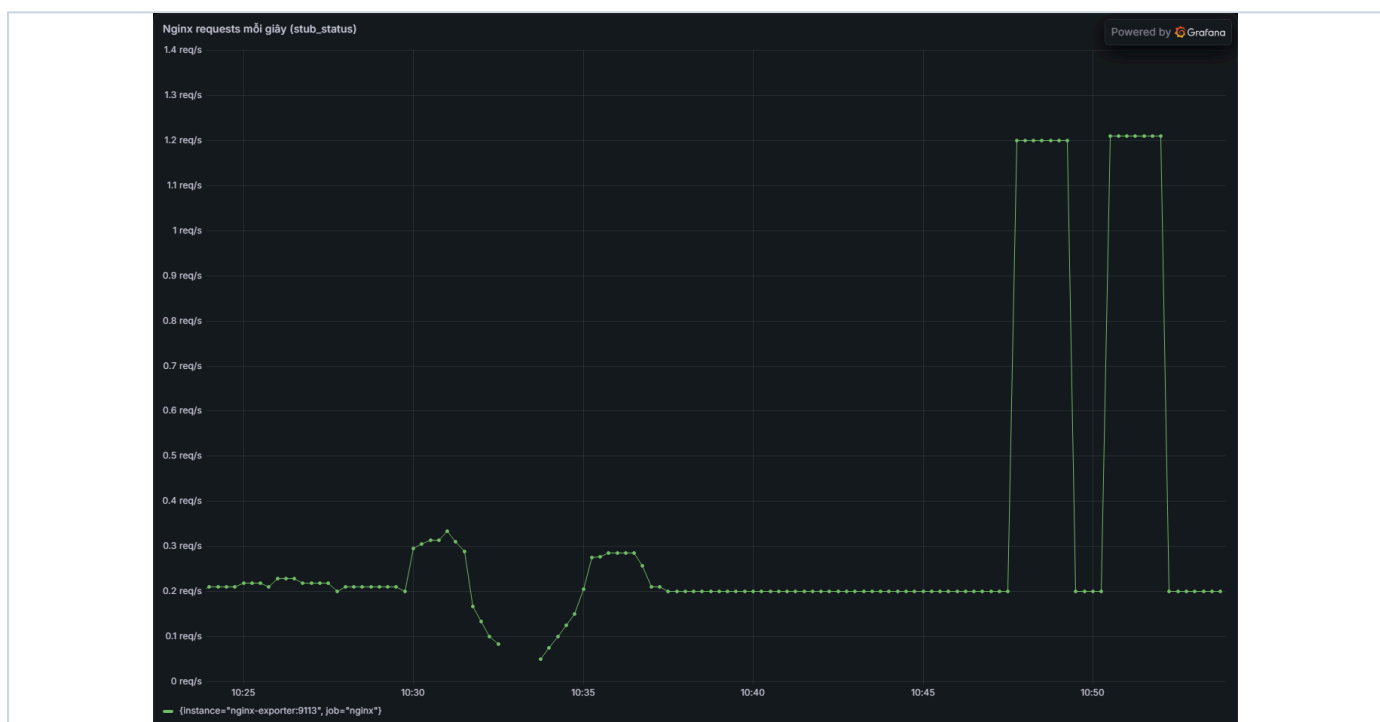
Hình 11. Panel Nginx requests/giây lấy từ nginx_http_requests_total.
