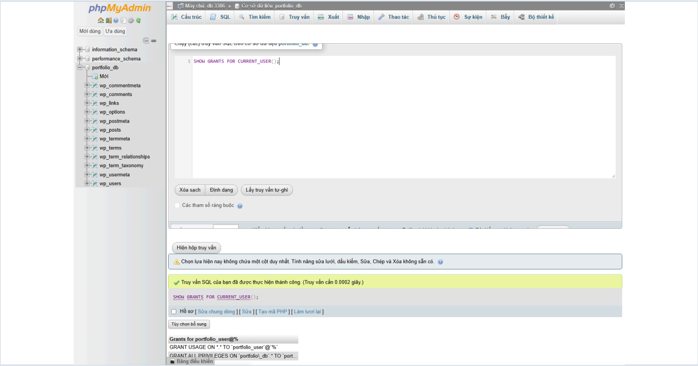
Hình 6. SHOW GRANTS FOR CURRENT_USER(): user portfolio_user có quyền trên schema portfolio_db. Chụp: 2026-10-08T10:56:14+07:00.
