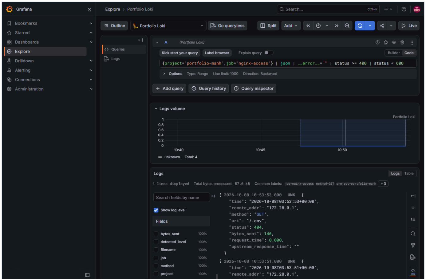
Hình 17. Grafana Explore: lọc numeric status 400–599, với request /.env trả 404 và /xmlrpc.php trả 403.
