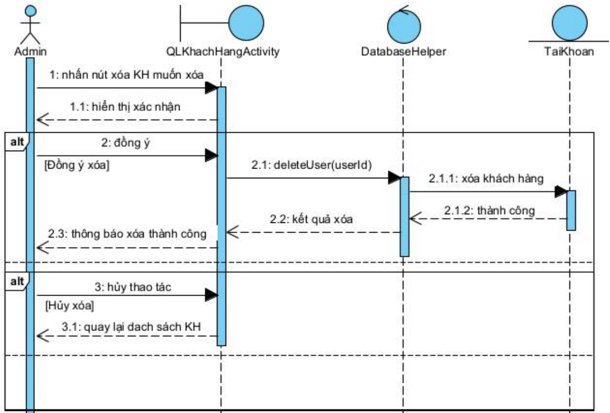
Hình 3 - 23: Biểu đồ tuần tự chức năng xóa khách hàng
