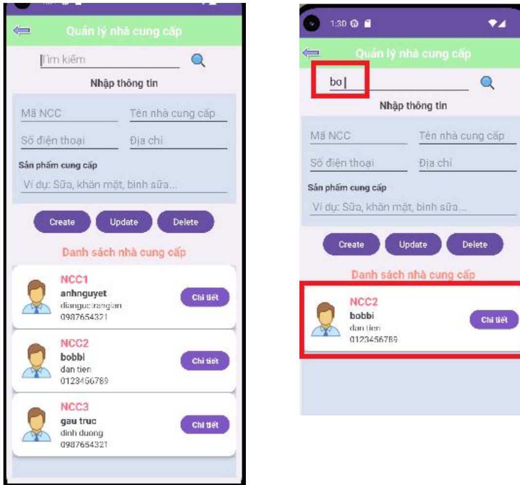
Hình 4 - 6: Triển khai chức năng tìm kiếm nhà cung cấp
