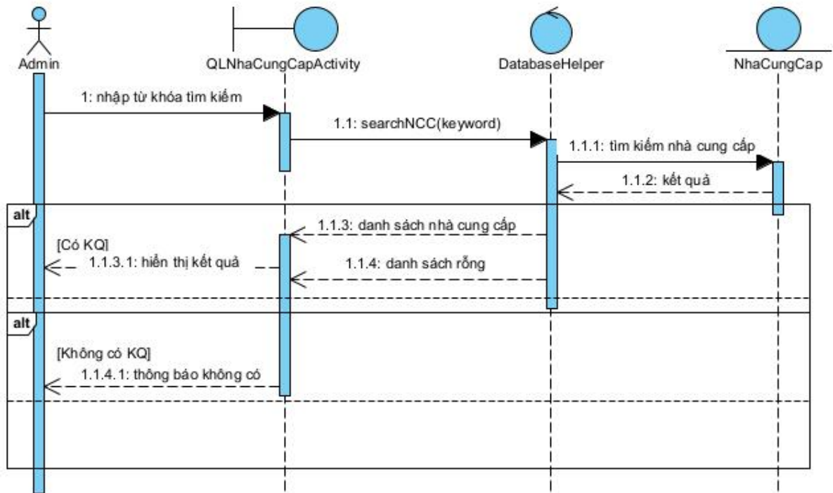
Hình 3 - 28: Biểu đồ tuần tự chức năng tìm kiếm nhà cung cấp
