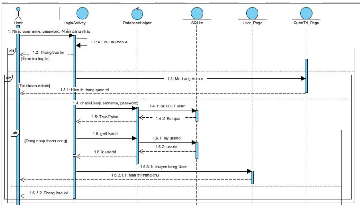
Hình 3 - 15: Biểu đồ tuần tự chức năng đăng nhập
