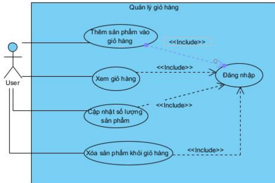
Hình 3 - 12: Biểu đồ use – case chức năng quản lý giỏ hàng
