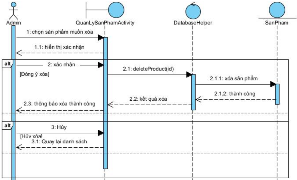
Hình 3 - 19: Biểu đồ tuần tự chức năng xóa sản phẩm
