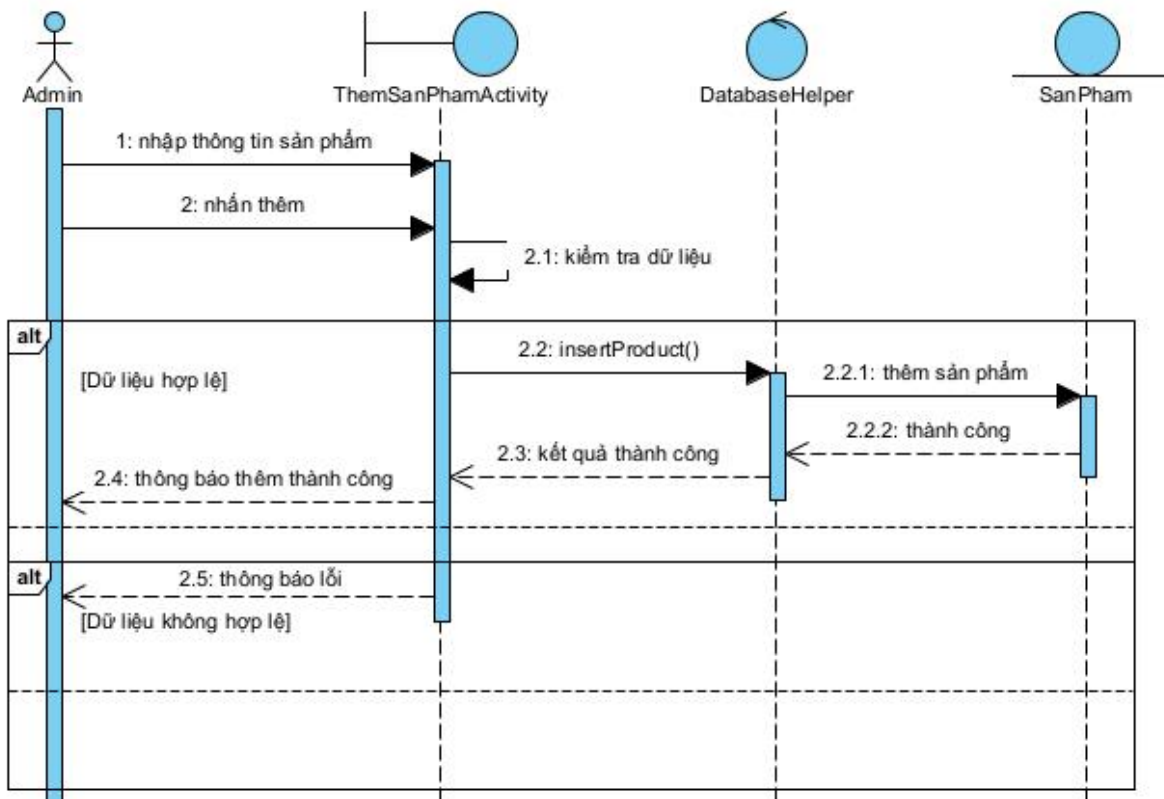
Hình 3 - 17: Biểu đồ tuần tự chức năng thêm sản phẩm
