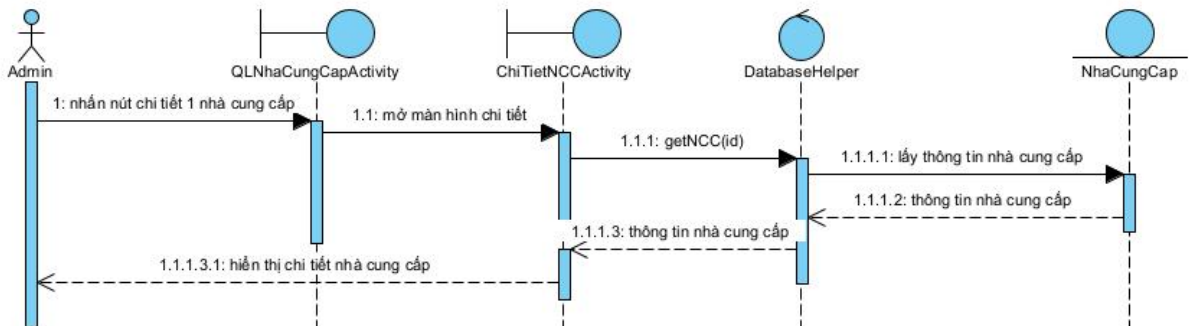
Hình 3 - 29: Biểu đồ tuần tự chức năng xem chi tiết nhà cung cấp
