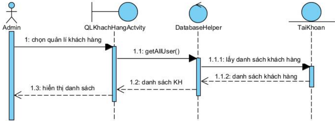
Hình 3 - 21: Biểu đồ tuần tự xem danh sách khách hàng
