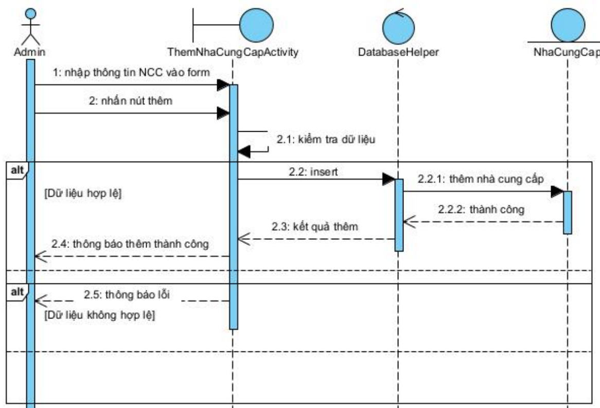
Hình 3 - 25: Biểu đồ tuần tự chức năng thêm nhà cung cấp
