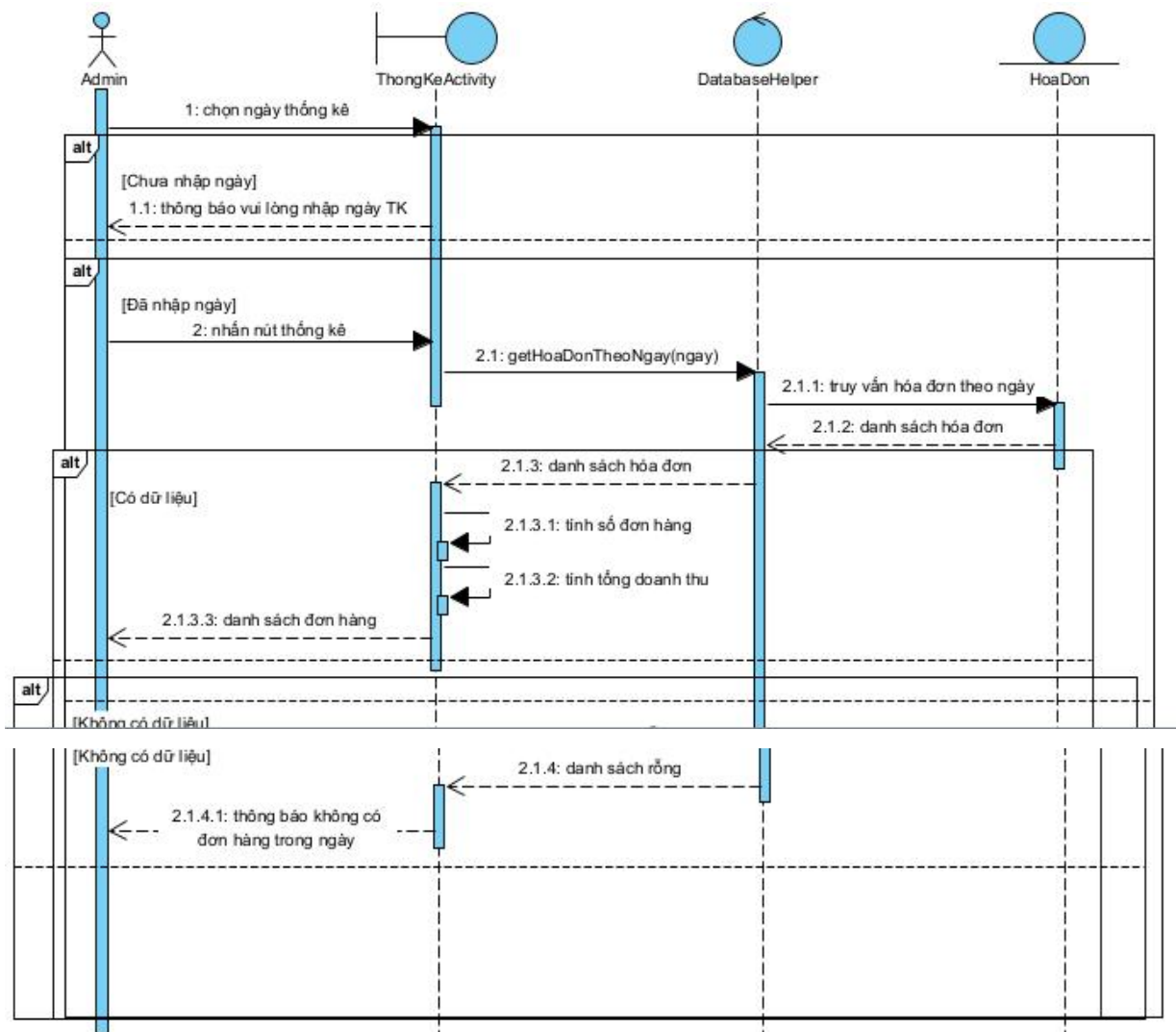
Hình 3 - 34: Biểu đồ tuần tự chức năng thống kê
