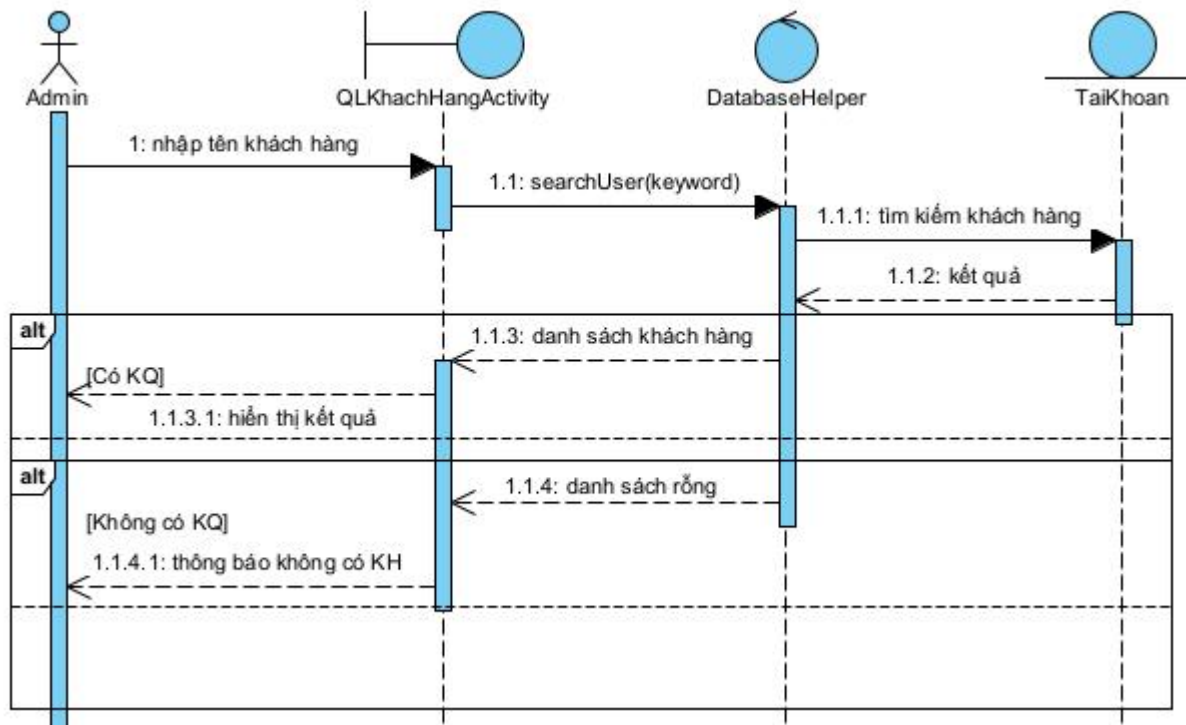
Hình 3 - 24: Biểu đồ tuần tự chức năng tìm kiếm khách hàng
