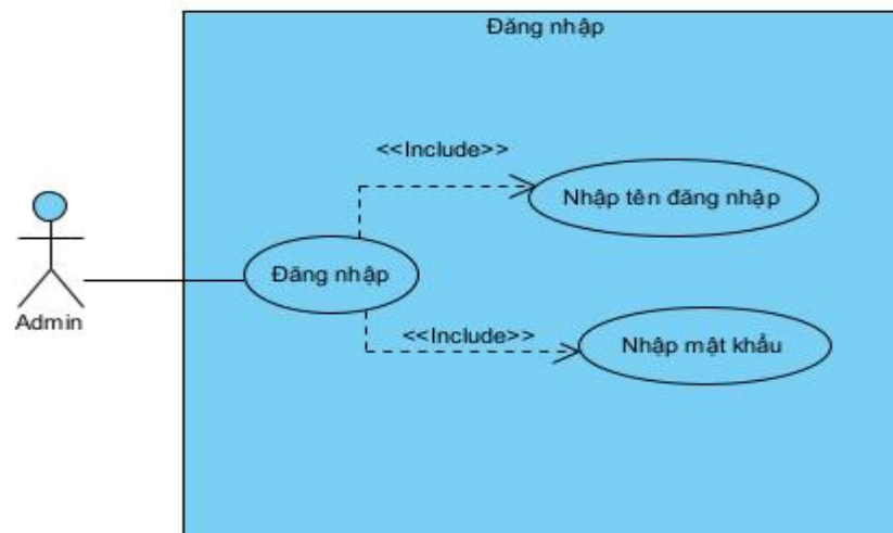
Hình 3 - 2: Biểu đồ use - case chức năng Admin đăng nhập
