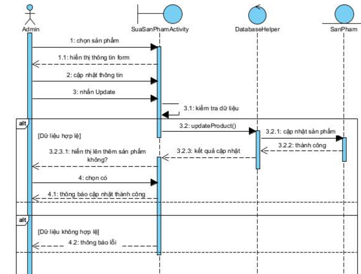
Hình 3 - 18: Biểu đồ tuần tự chức năng sửa sản phẩm
