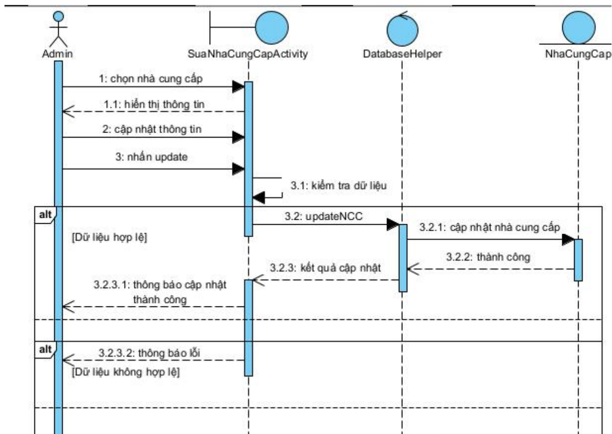
Hình 3 - 26: Biểu đồ tuần tự chức năng cập nhật nhà cung cấp
