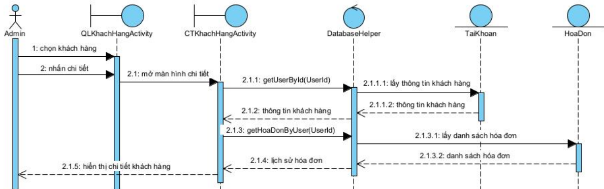
Hình 3 - 22: Biểu đồ tuần tự chức năng xem chi tiết khách hàng
