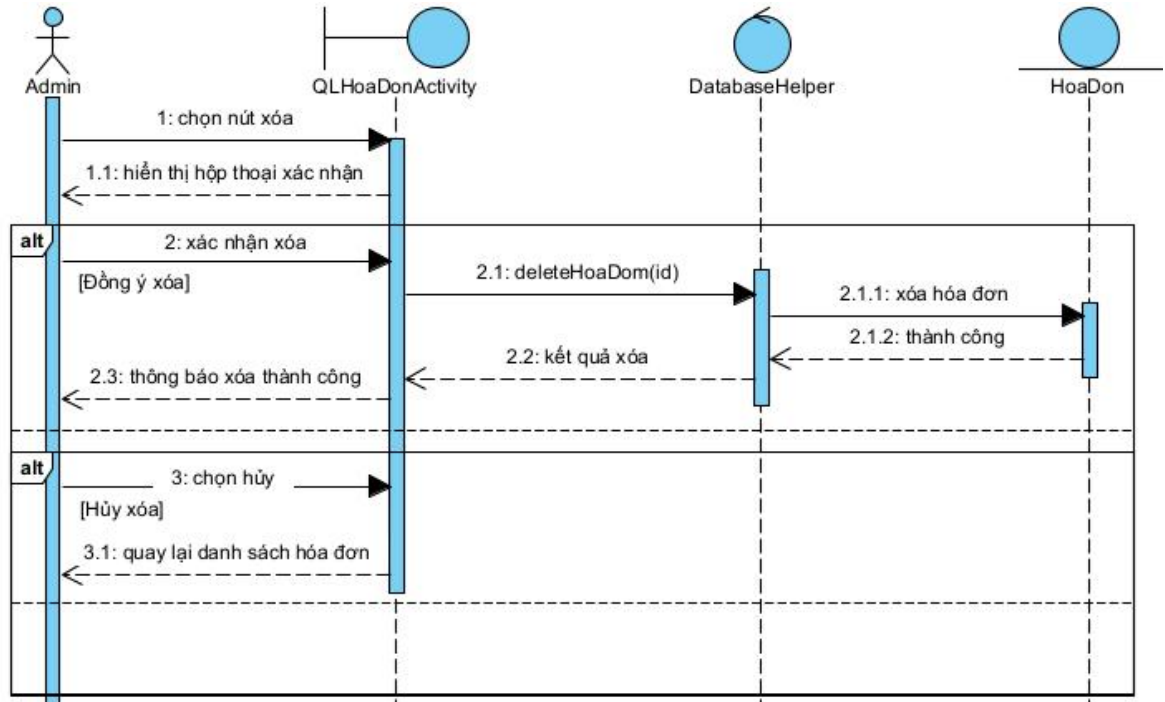
Hình 3 - 32: Biểu đồ tuần tự chức năng xóa hóa đơn
