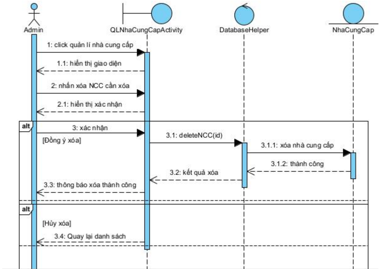
Hình 3 - 27: Biểu đồ tuần tự chức năng xóa nhà cung cấp
