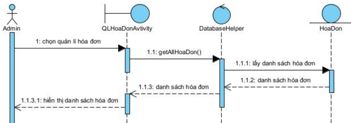
Hình 3 - 30: Biểu đồ tuần tự xem danh sách hóa đơn
