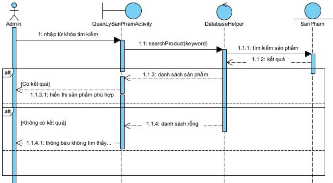
Hình 3 - 20: Biểu đồ tuần tự chức năng tìm kiếm sản phẩm
