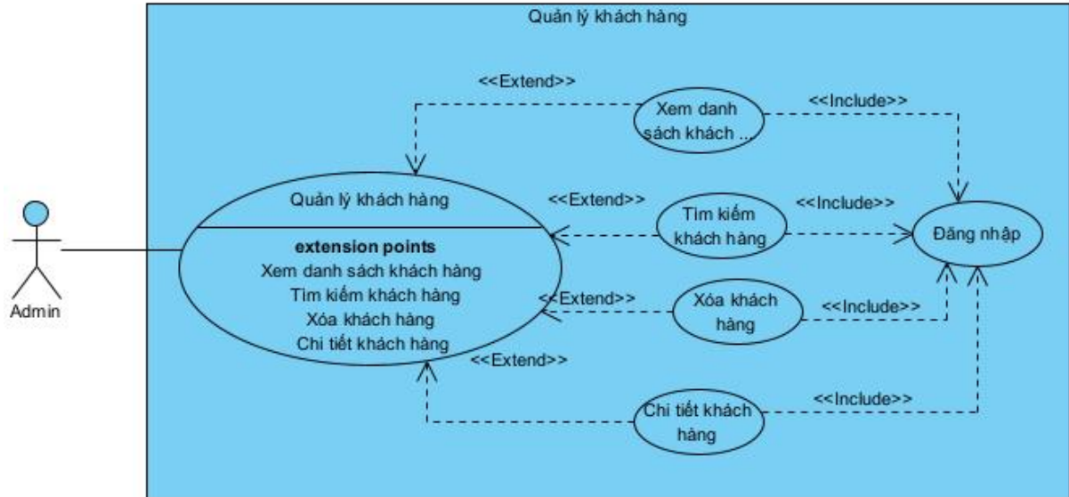
Hình 3 - 4: Biểu đồ use – case chức năng quản lý khách hàng
