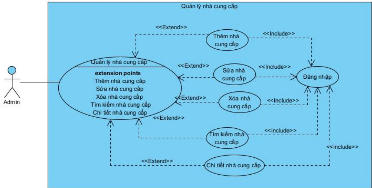
Hình 3 - 5: Biểu đồ use – case chức năng quản lý nhà cung cấp
