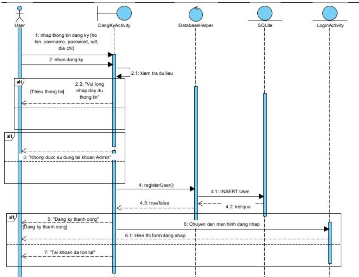
Hình 3 - 16: Biểu đồ tuần tự chức năng đăng ký
