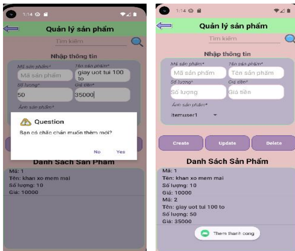
Hình 4 - 4: Triển khai chức năng thêm sản phẩm
