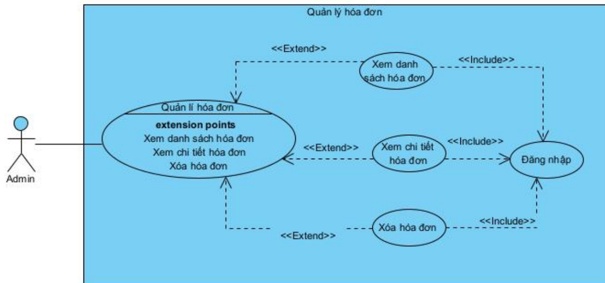
Hình 3 - 6: Biểu đồ use case chức năng quản lý hóa đơn
