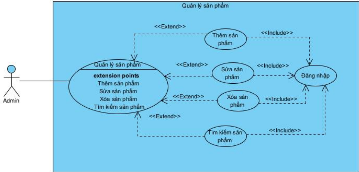
Hình 3 - 3: Biểu đồ use – case chức năng quản lý sản phẩm
