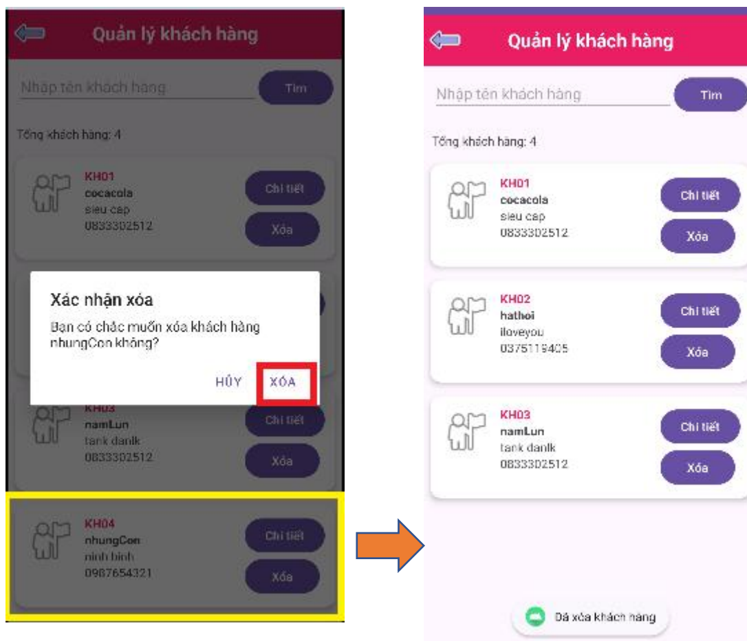
Hình 4 - 5: Triển khai chức năng xóa khách hàng
