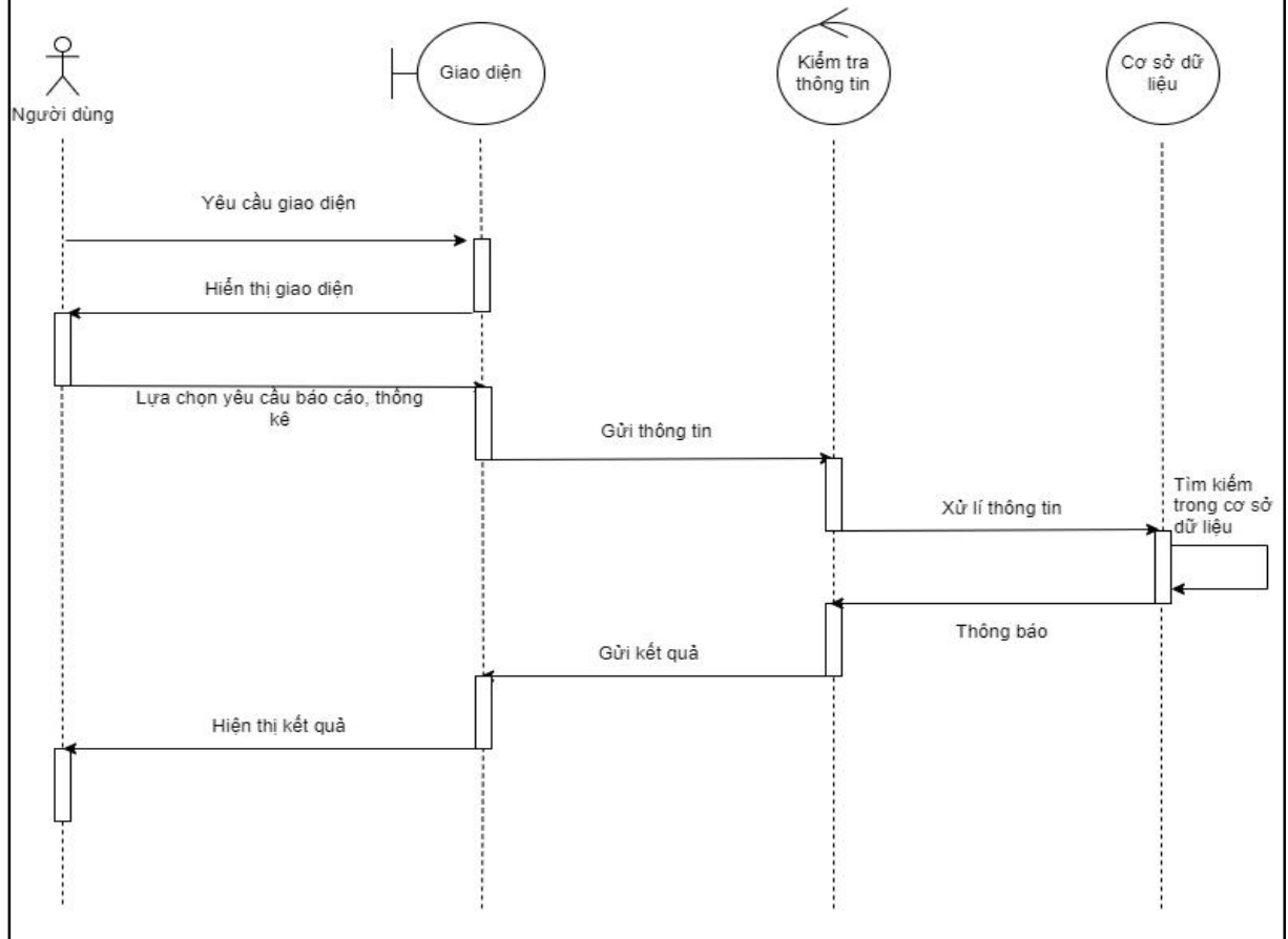
Biểu đồ tuần tự chức năng báo cáo thống kê
