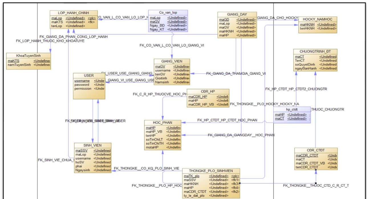
Hình 3.2 Mô hình dữ liệu vật lý
