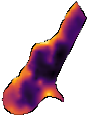
Predição (Log Zinc)
