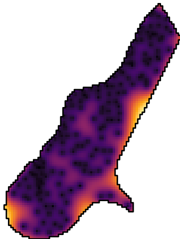
Variância de Krigagem
