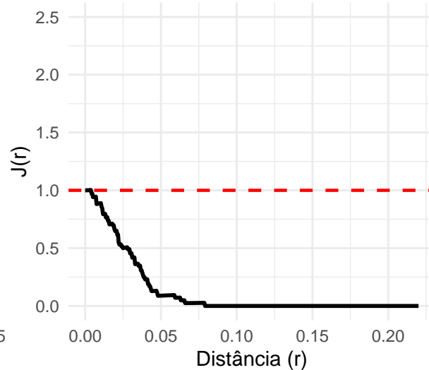
(c) Agrupado J(r) < 1 (Atração)
