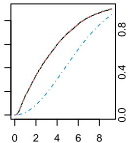
Função g (PCF)
