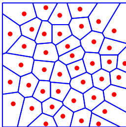
Voronoi
