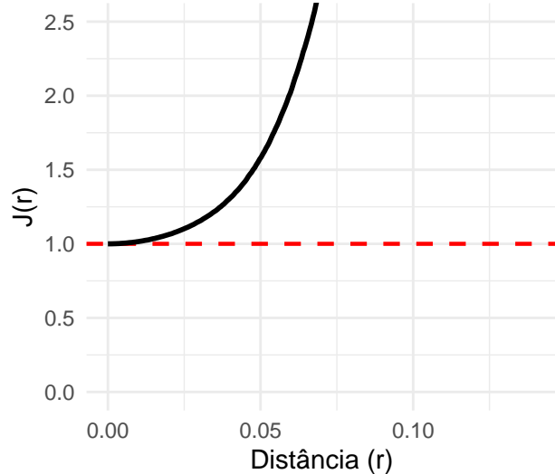
(a) Regular J(r) > 1 (Inibição)
