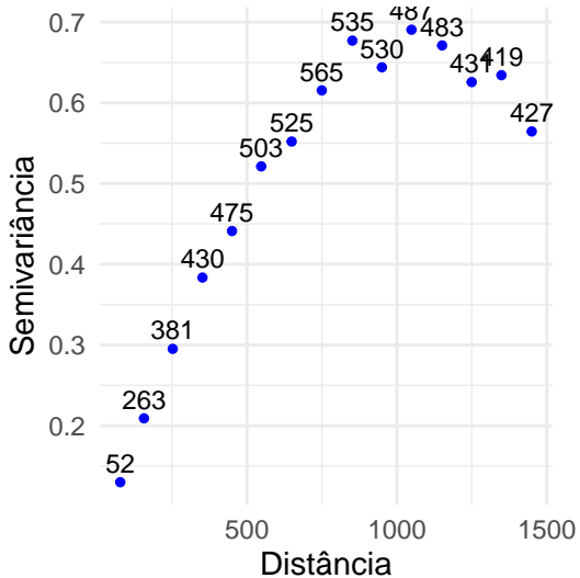
Variograma Experimental (M Números indicam pares por lag
