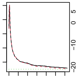
Função g (PCF)
