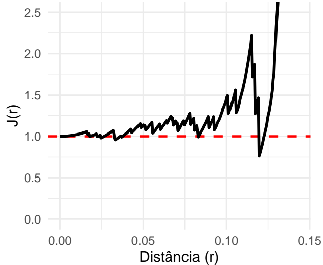
(b) Aleatório J(r) = 1 (Independência)
