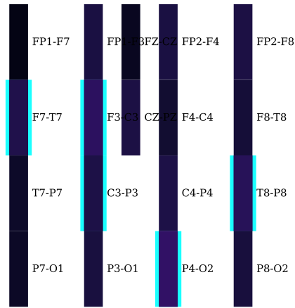
chb06 [---] LI=-0.06
