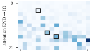
Pythia-410M
