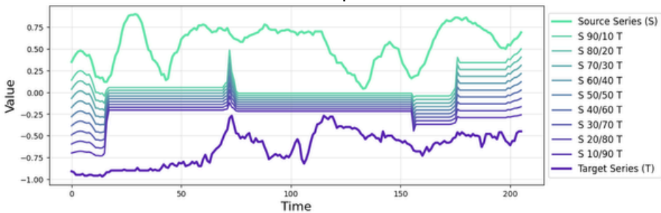
DBA Morph
