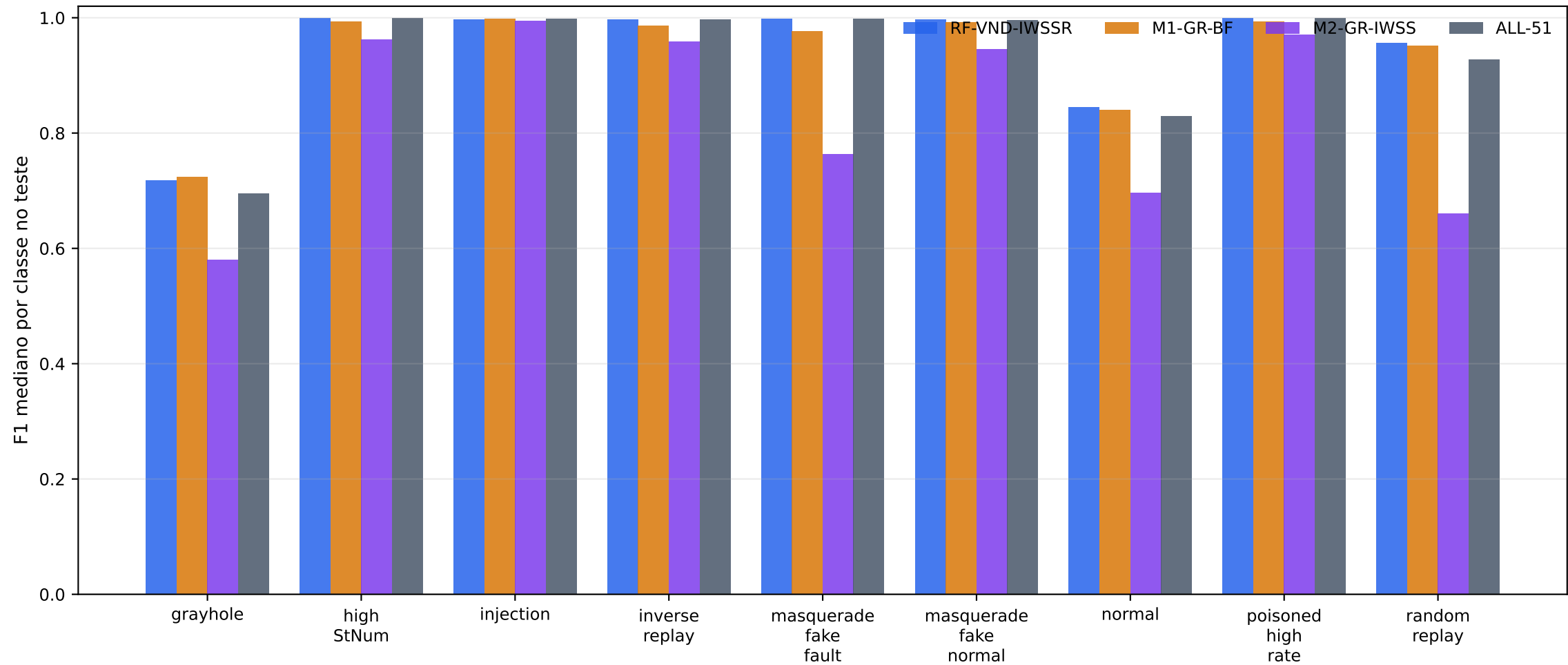
Desempenho por classe da configuração G-FShield escolhida na validação e dos comparadores
