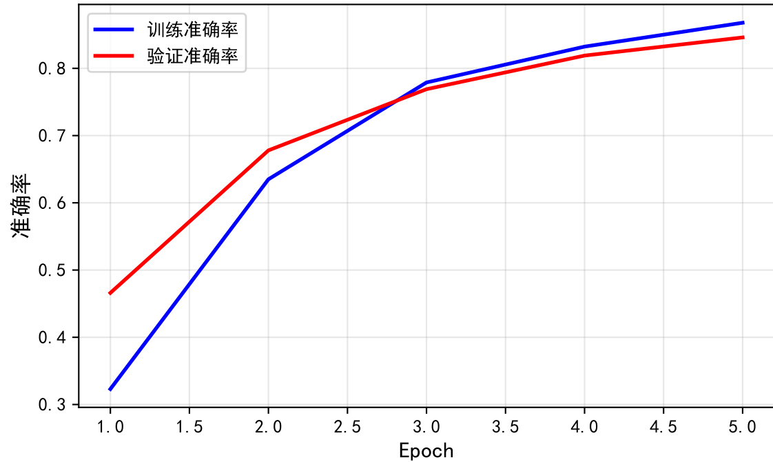
训练和验证准确率
