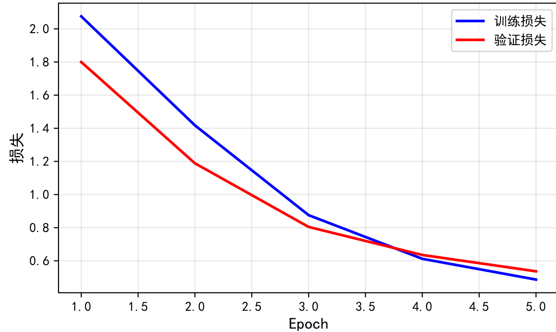
训练和验证损失
