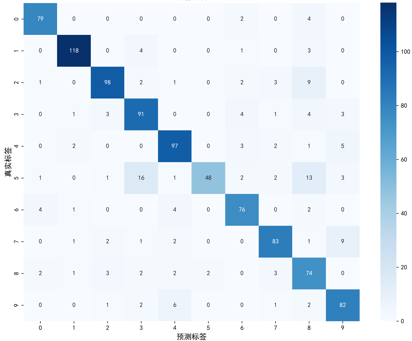
混淆矩阵
