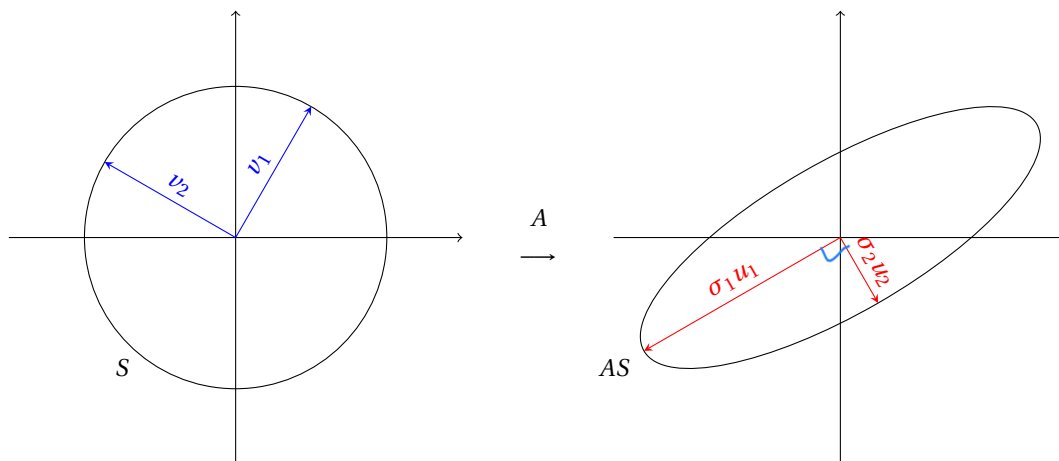
Figura A.1: SVD de una matriz 2 \times 2
