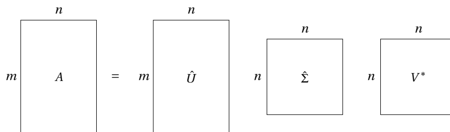
Figura A.2: Factorización SVD reducida.
