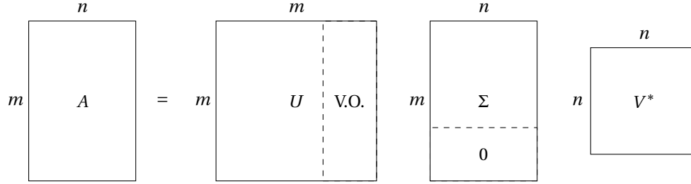
Figura A.3: Factorización SVD completa.
