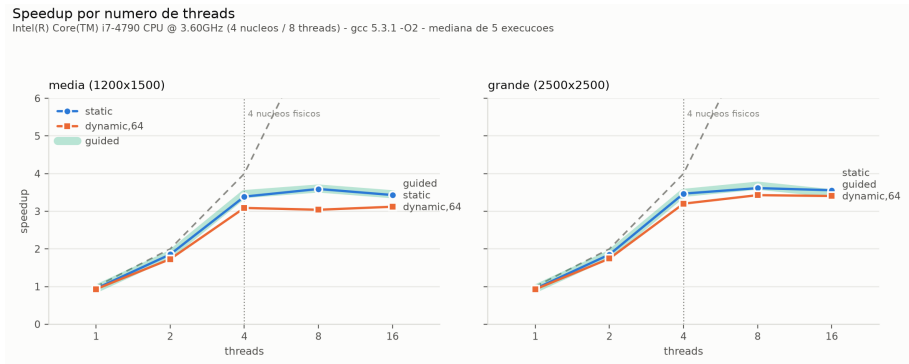
Figura 1. Speedup em função do número de threads. A linha tracejada cinza marca o speedup linear ideal e a pontilhada vertical marca o limite de núcleos físicos. As curvas de static e guided são praticamente coincidentes, por isso guided aparece como faixa larga sob a linha de static .
