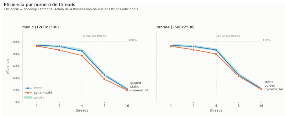
Figura 2. Eficiência em função do número de threads.
