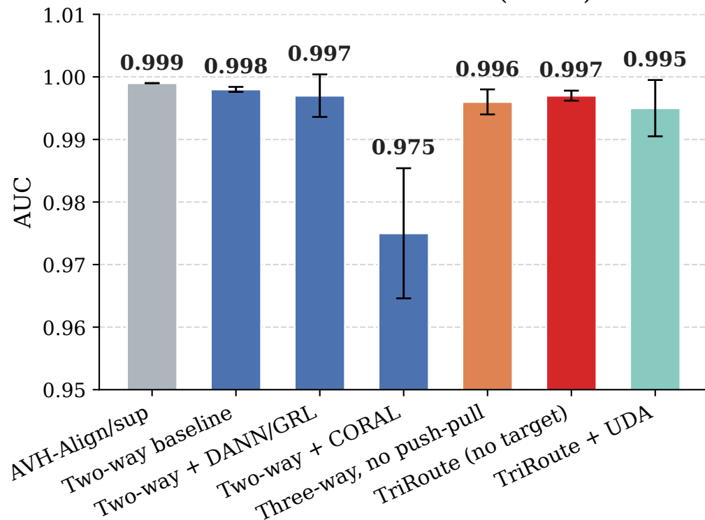
FakeVideo-FakeAudio (FV-FA)
