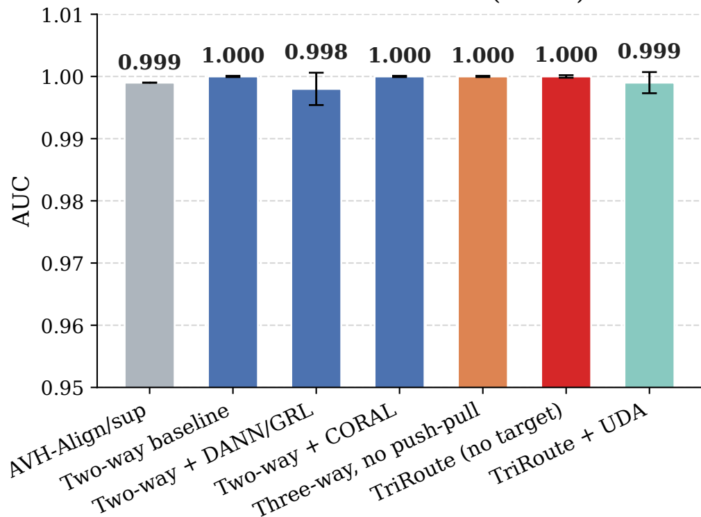
RealVideo-FakeAudio (RV-FA)
