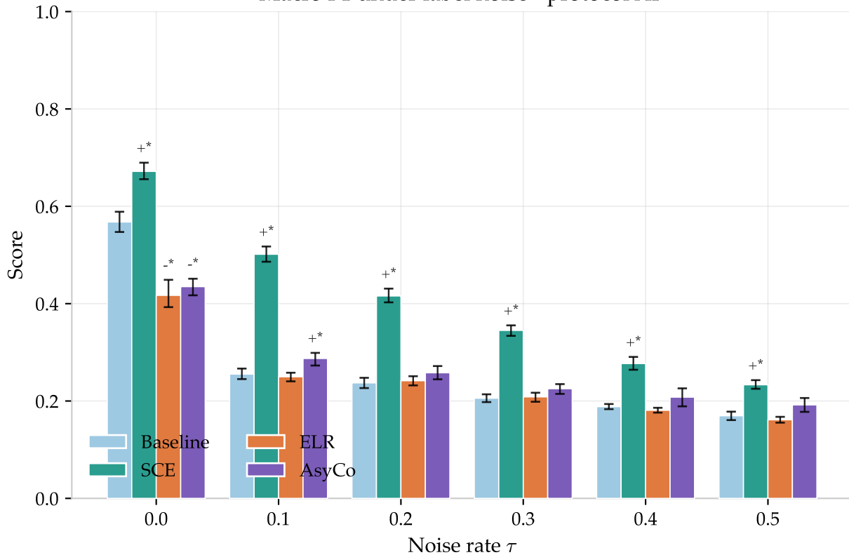
Macro F1 under label noise - protocol AP
