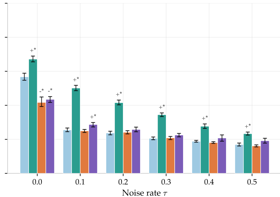
Macro F1
