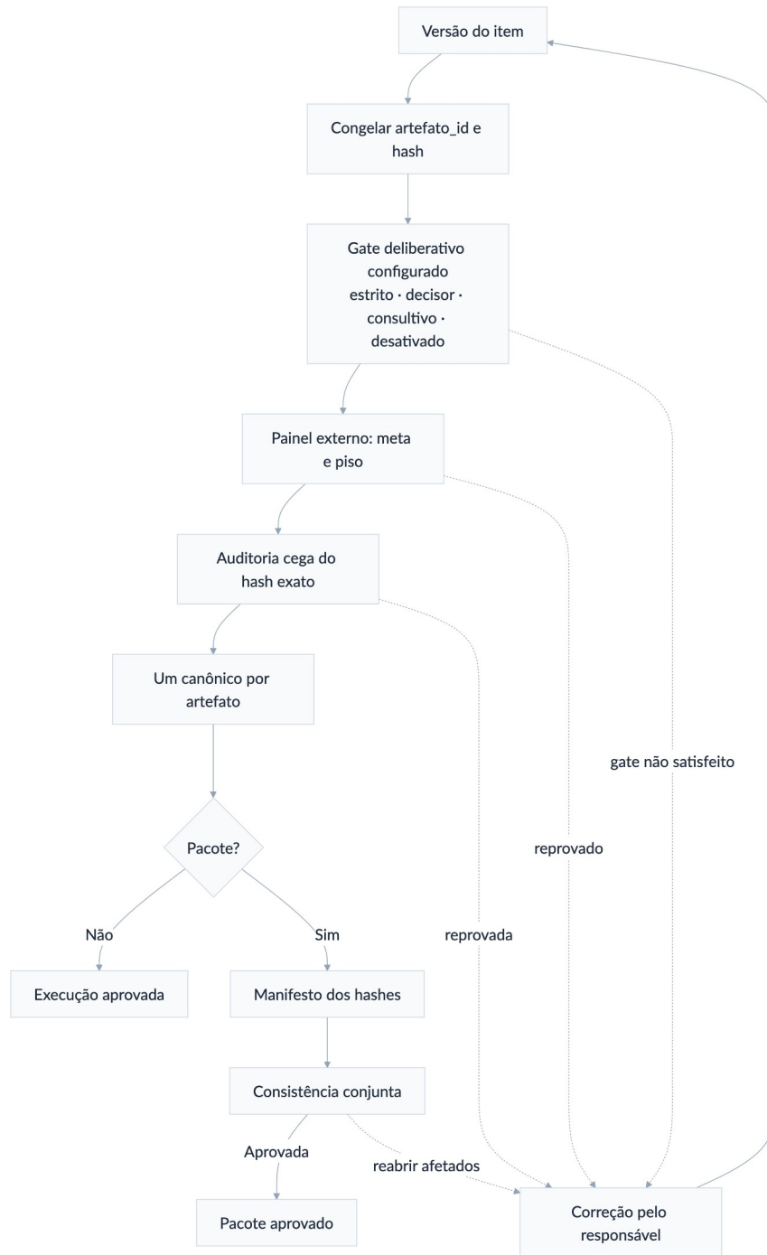
Figura 7 – Debate, correção e novo consenso sobre cada versão do artefato.
