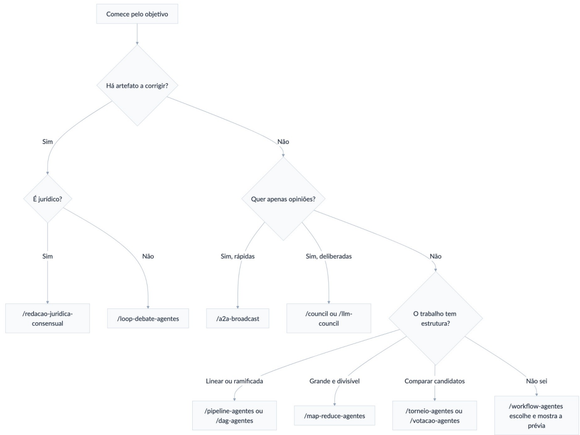
Figura 2 – Árvore de escolha do comando conforme a finalidade do trabalho.
