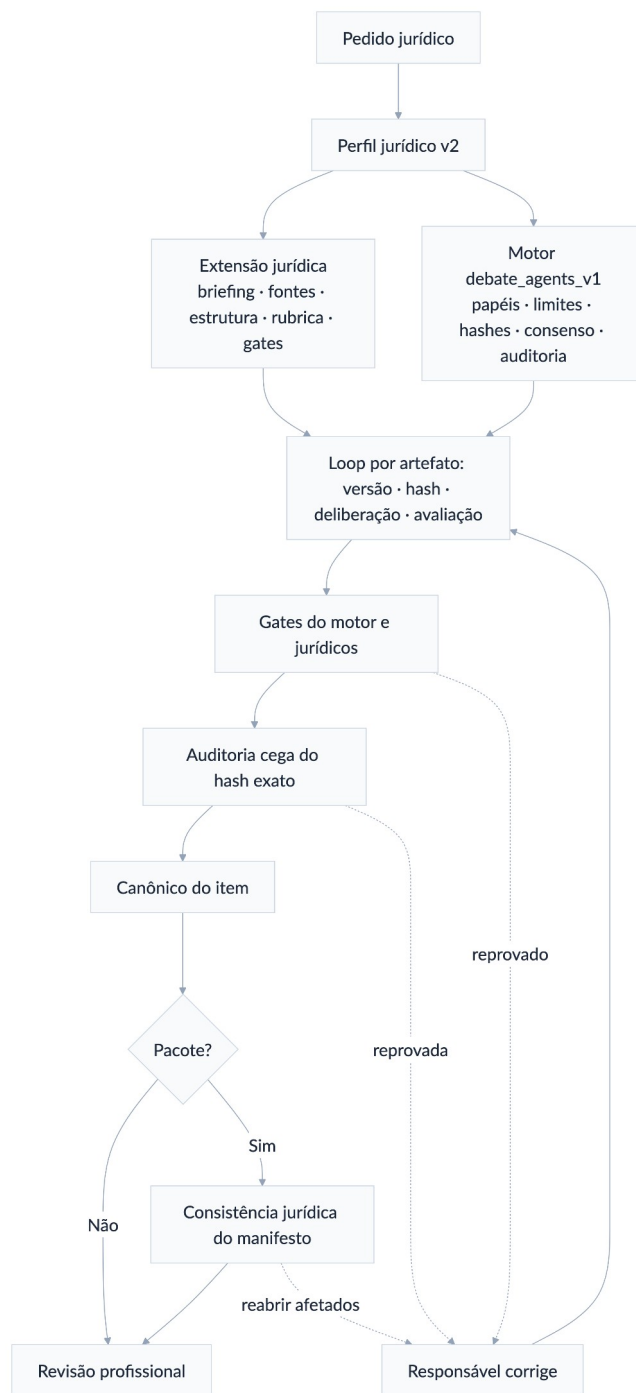
Figura 10 – Fluxo integral da redação jurídica consensual e de seus artefatos.
