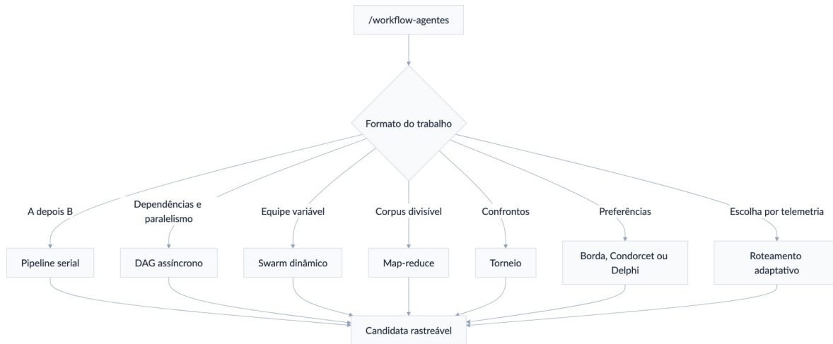
Figura 11 – Protocolos formais disponíveis para organizar o trabalho multiagente.
