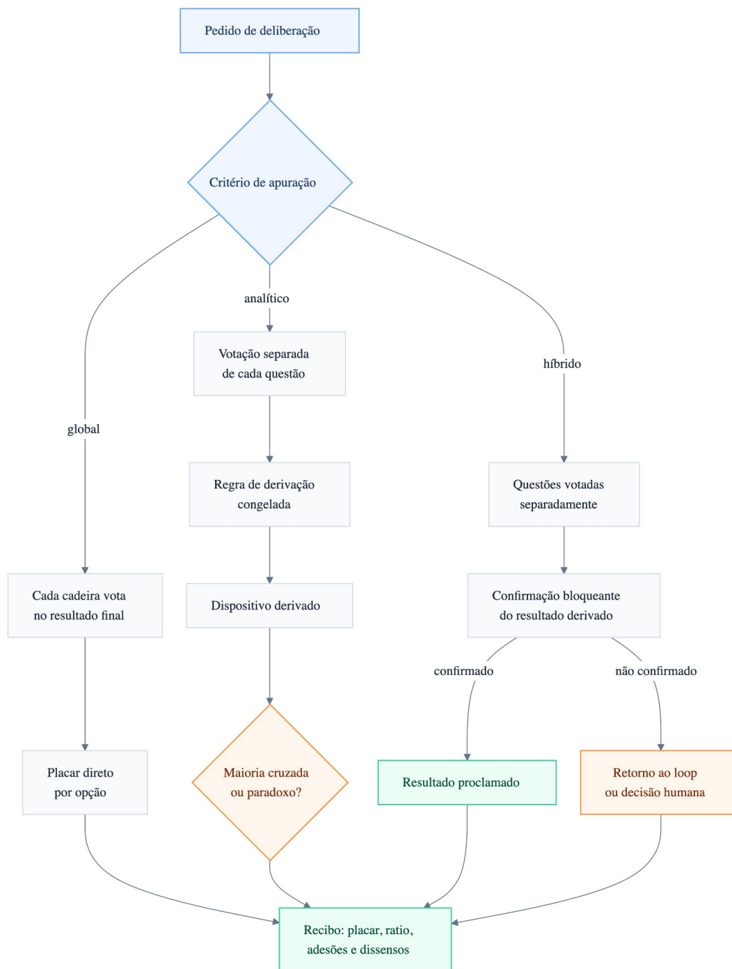
Figura 3 – Critérios global, analítico e híbrido para apuração colegiada.
