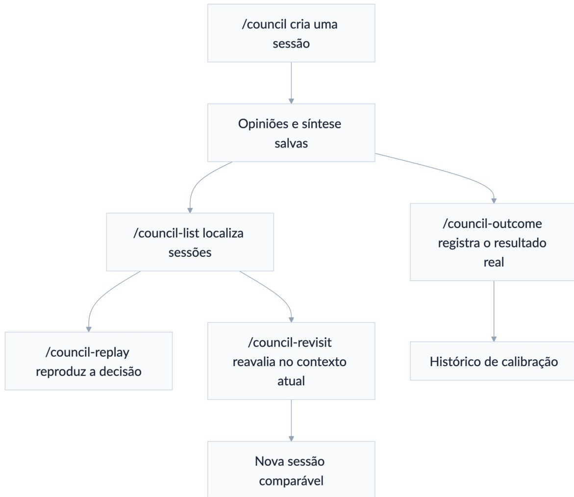
Figura 12 – Persistência, retomada, replay e encerramento de sessões do Council.
