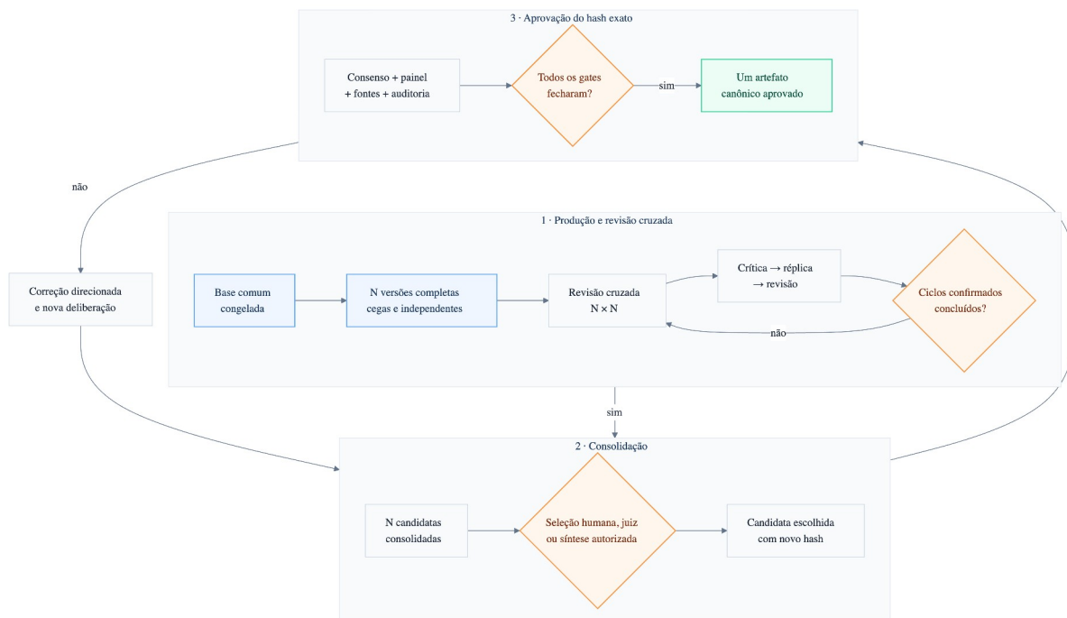
Figura 9 – Produção independente, revisão cruzada, consolidação e gates finais.
