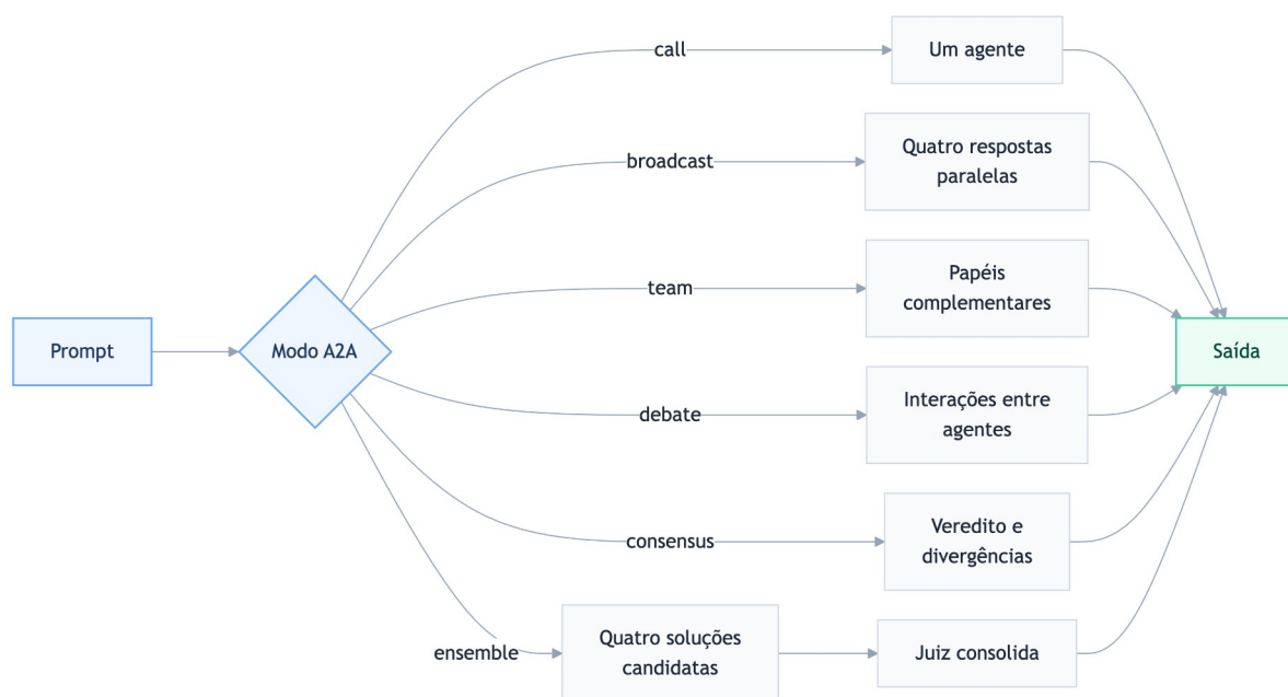
Figura 6 – Modos de convocação e colaboração disponíveis no A2A Mesh.
