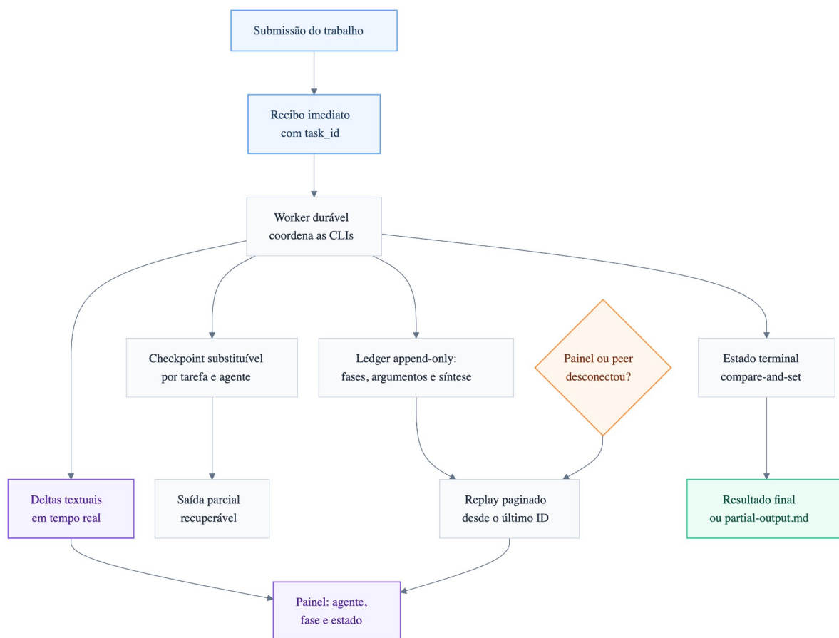
Figura 5 – Separação entre streaming ao vivo, ledger durável, replay e recuperação.
