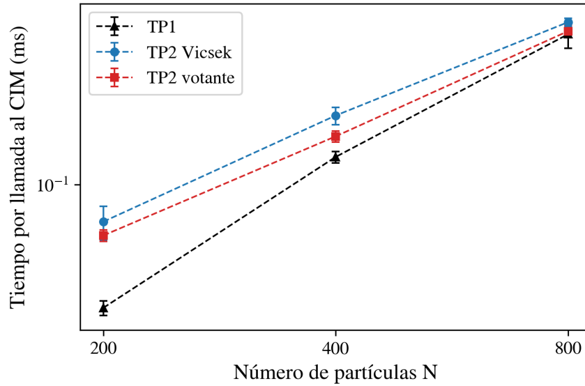
Figura 15: Tiempo por llamada al CIM en función de la cantidad de partículas, para el bench del TP1 y para ambos modelos del TP2. Geometría común: L = 10 m, M = 10 , r_c = 1 m, condiciones periódicas y partículas puntuales. Las barras son desvíos estándar y las rectas, guías para el ojo.
