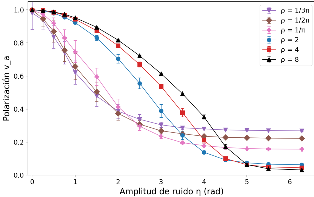
Figura 3: Polarización estacionaria en función del ruido para el modelo de Vicsek. Cada punto es el promedio de 50 realizaciones y las barras representan el desvío estándar muestral. Las rectas son guías para el ojo. Además de las densidades exigidas se muestran tres densidades complementarias.
