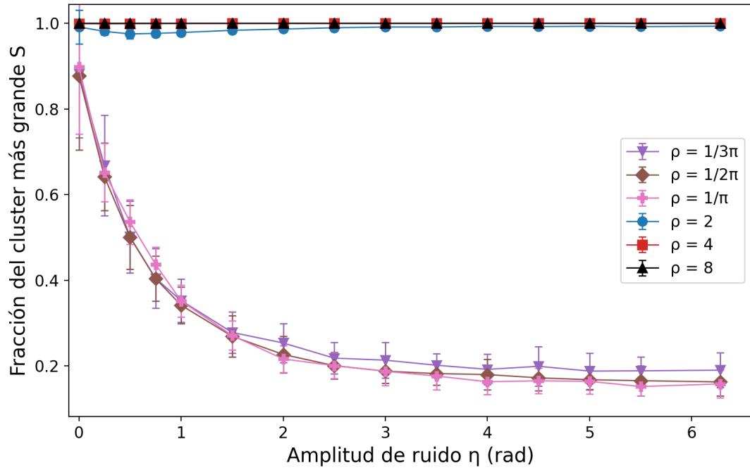
Figura 11: Fracción estacionaria del cluster más grande en función del ruido para el modelo de votante. Cada punto promedia 50 realizaciones; las barras son desvíos estándar y las rectas, guías para el ojo.
