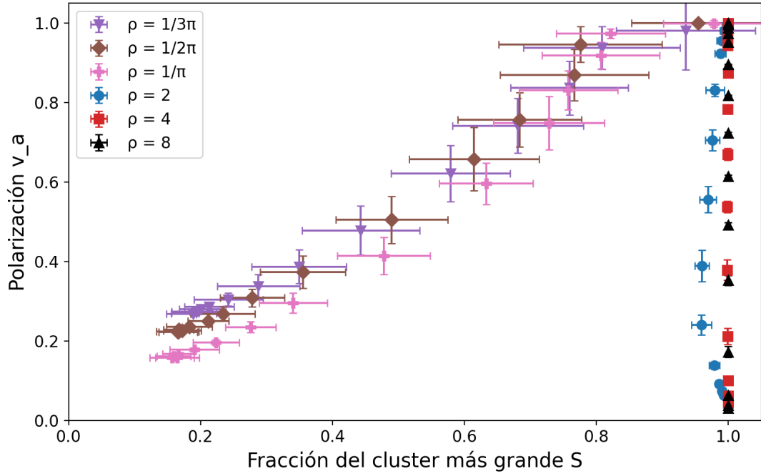
Figura 6: Polarización en función de la fracción del cluster más grande para Vicsek. Cada punto corresponde a un valor de ruido; las barras horizontales y verticales son los desvíos estándar de S y v_a , respectivamente.
