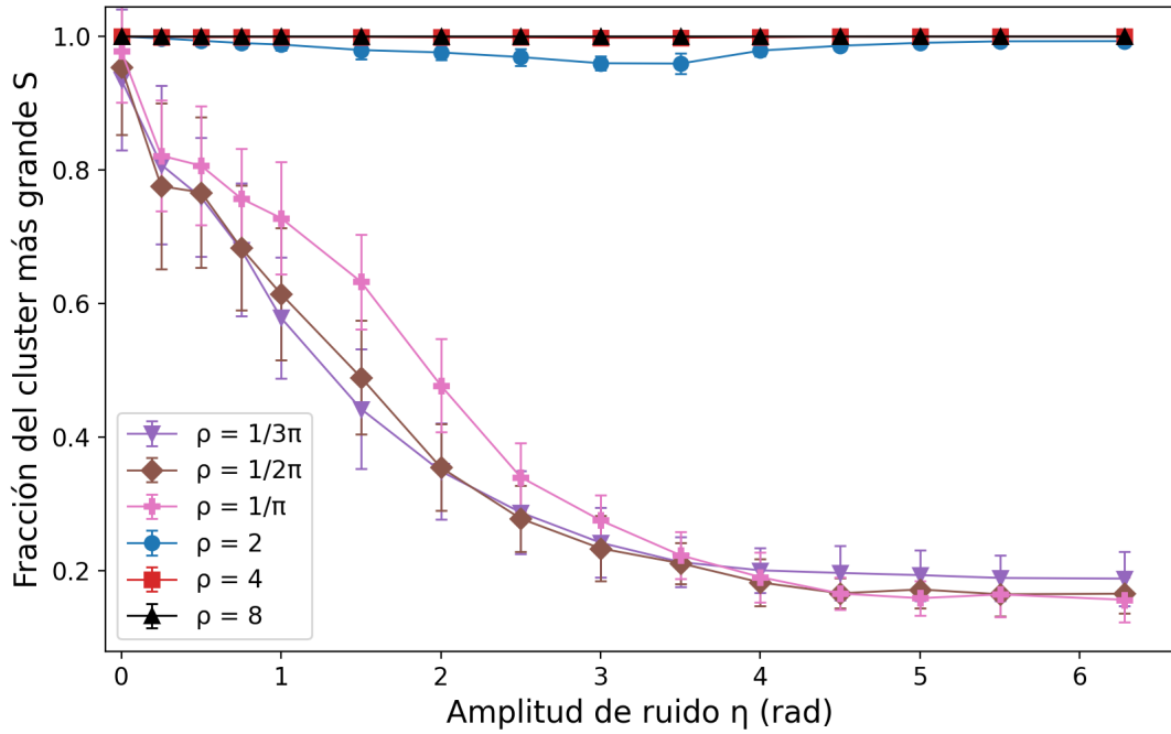
Figura 5: Fracción estacionaria del cluster más grande en función del ruido para el modelo de Vicsek. Cada punto promedia 50 realizaciones; las barras son desvíos estándar y las rectas, guías para el ojo.
