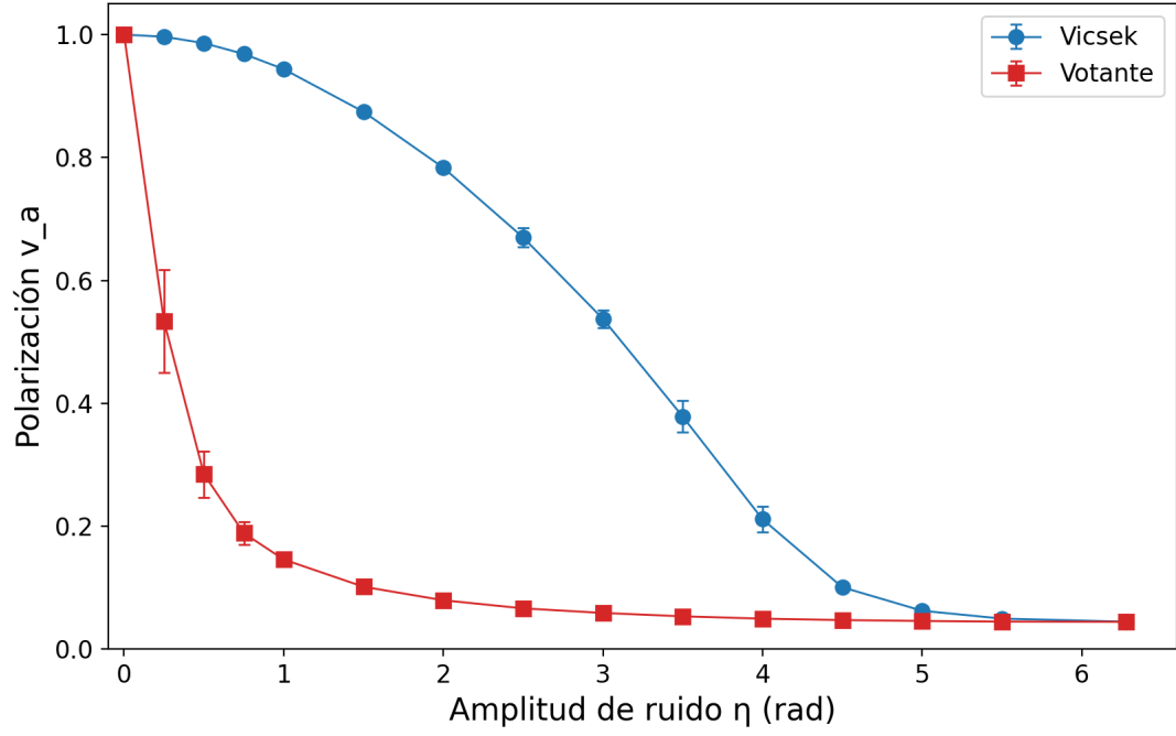
Figura 9: Polarización estacionaria en función del ruido para Vicsek y votante con \rho = 4 . Cada punto promedia 50 realizaciones y las barras representan el desvío estándar muestral. Las rectas son guías para el ojo.
