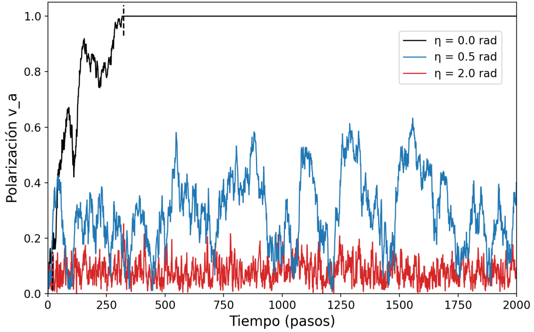
Figura 8: Evolución de la polarización en el modelo de votante para \rho = 4 ( N = 400 ) y una realización representativa. La ausencia de una marca vertical para \eta = 0,5 rad indica que la realización seleccionada no alcanza un plateau estrecho. Parámetros fijos: L = 10 m, r_c = 1 m, v = 0,03 m/s y \Delta t = 1 s.
