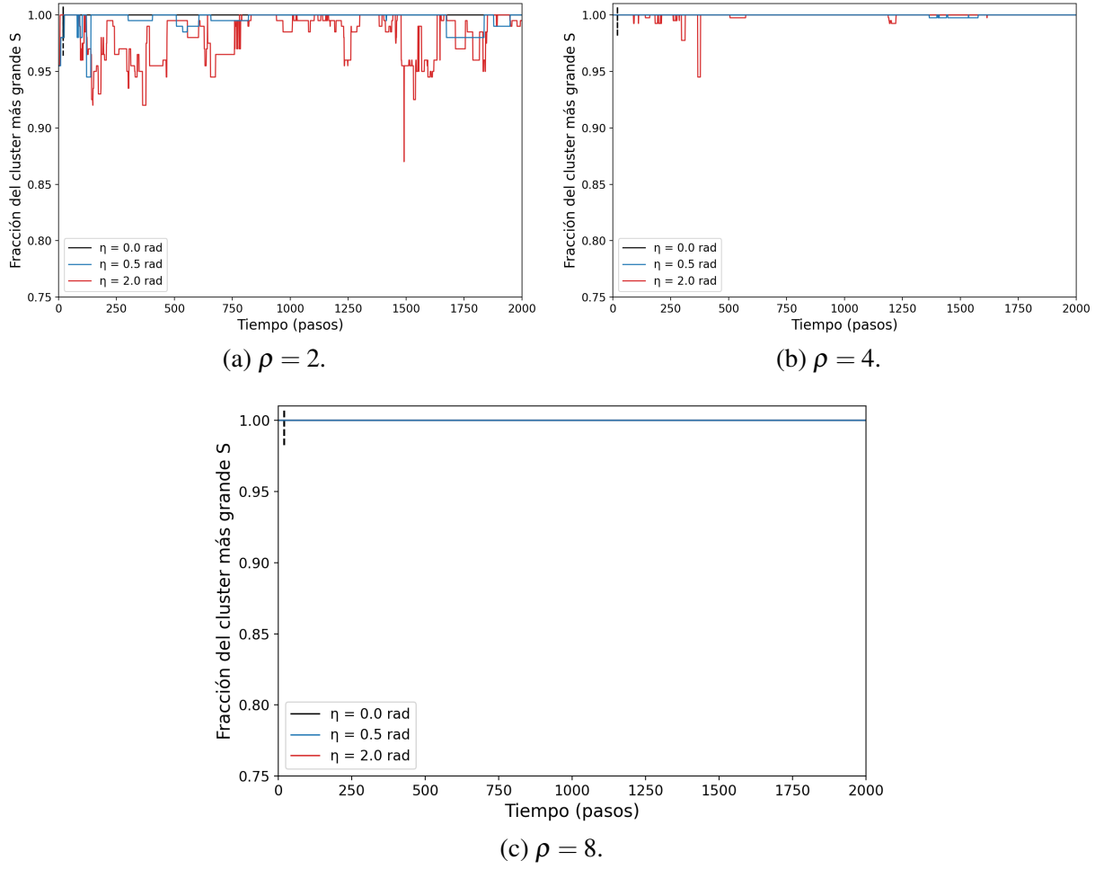
Figura 4: Evolución de la fracción del cluster más grande para Vicsek y las tres densidades exigidas. Cada panel corresponde a una realización y compara \eta = 0, 0,5 y 2 rad. Los ejes verticales se acotaron al intervalo donde varían los datos.
