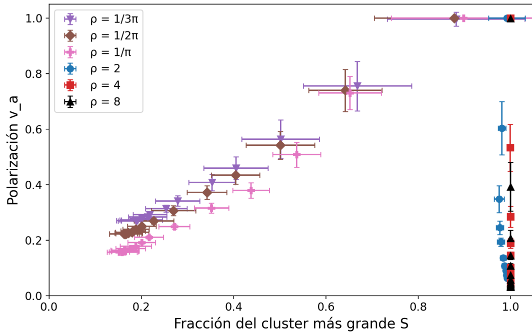
Figura 12: Polarización en función de la fracción del cluster más grande para el votante. Cada punto corresponde a un valor de ruido; las barras horizontales y verticales son los desvíos estándar de S y v_a , respectivamente.
