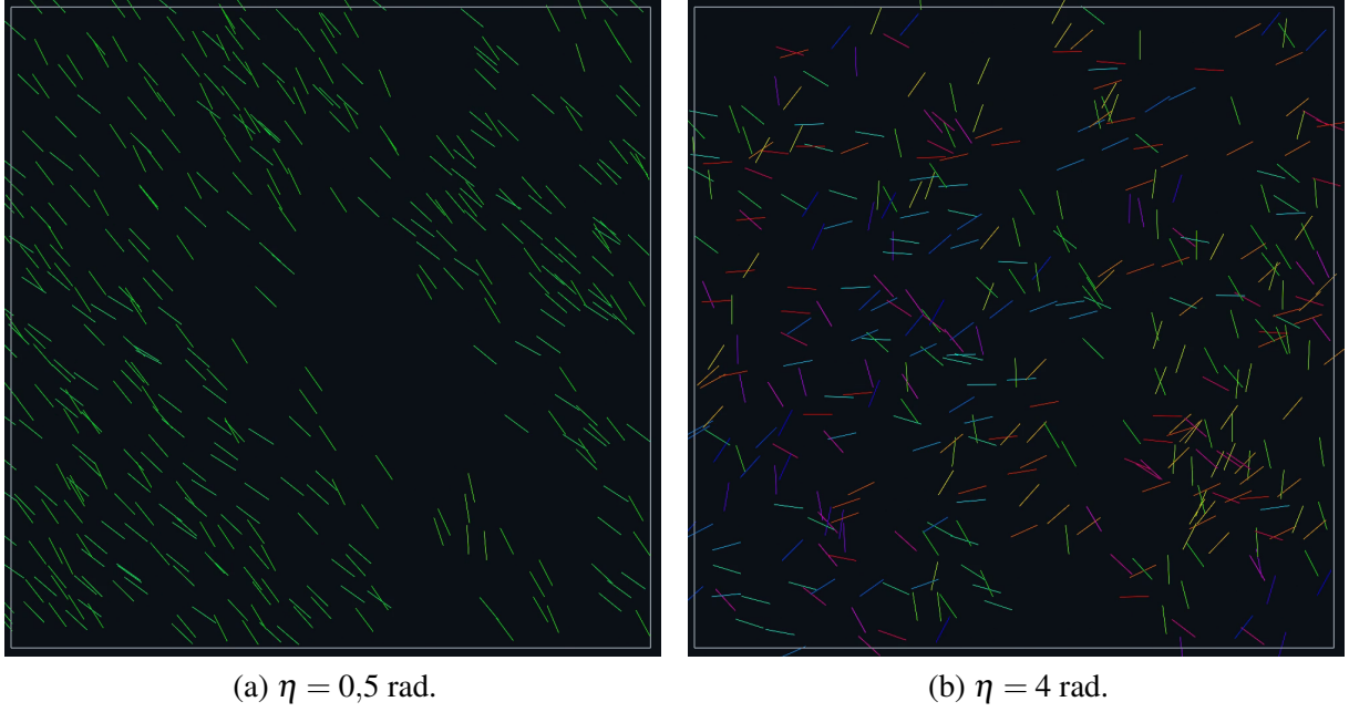
Figura 1: Fotografías en t = 1500 s de una realización del modelo de Vicsek para \rho = 4 ( N = 400 ), dentro de la ventana de promediado t \geq T/2 . Cada segmento representa la velocidad de una partícula y su color, el ángulo de movimiento. Parámetros fijos: L = 10 m, r_c = 1 m, v = 0,03 m/s y \Delta t = 1 s.
