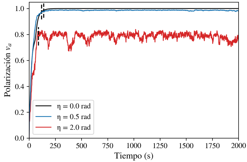
Figura 2: Evolución de la polarización en el modelo de Vicsek para \rho = 4 ( N = 400 ) y una realización representativa. Parámetros fijos: L = 10 m, r_c = 1 m, v = 0,03 m/s y \Delta t = 1 s.
