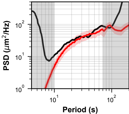
Vertical Seismic Displ.
