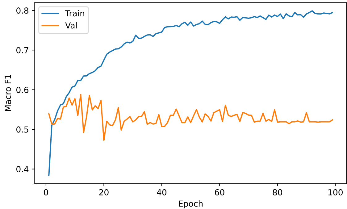
Macro F1 curves
