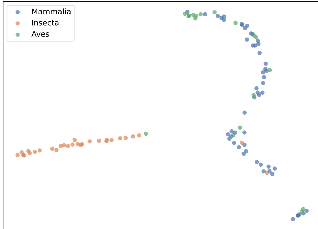
UMAP
