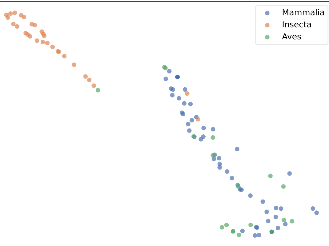
t-SNE
