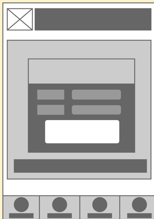
設定頁步驟2
