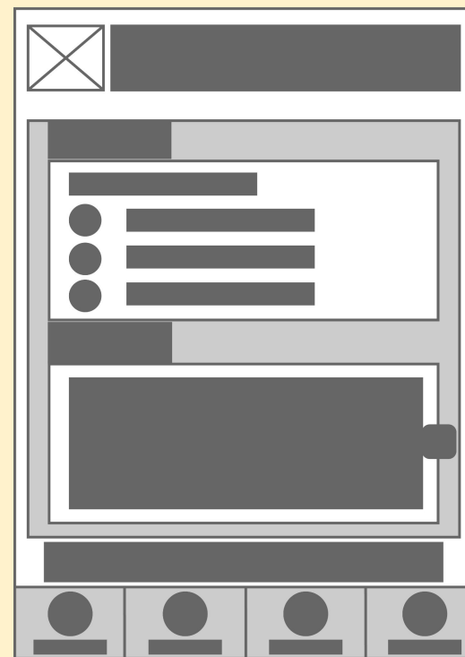
首頁2(右滑後)
