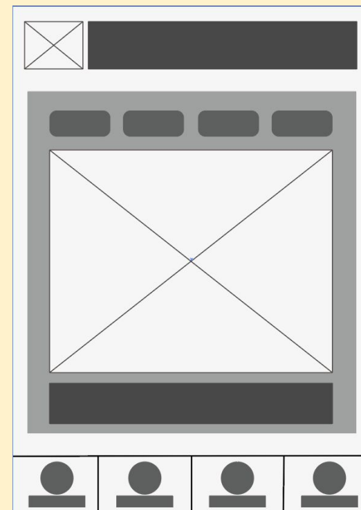
趨勢分析
