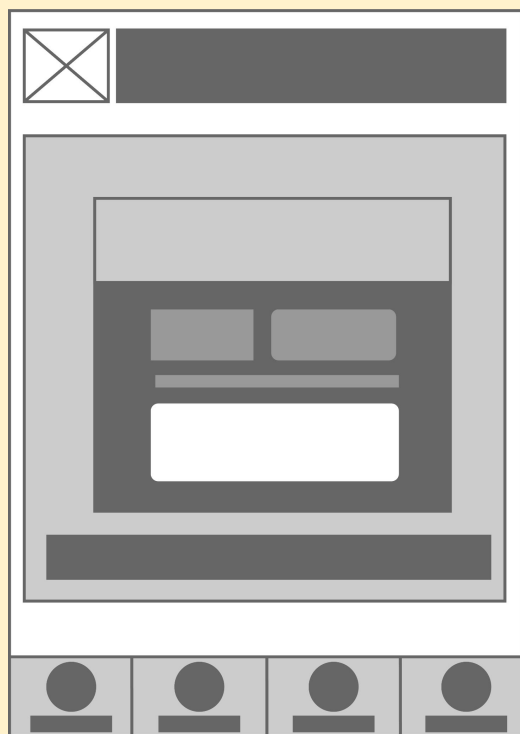
設定頁步驟4
