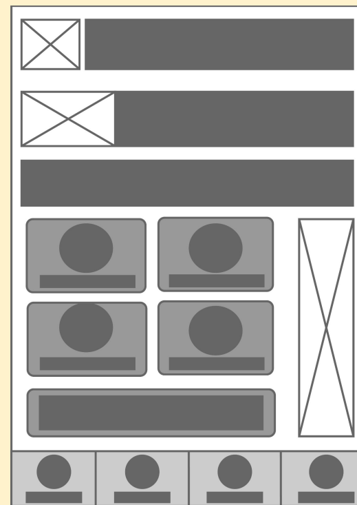
帳戶設定
