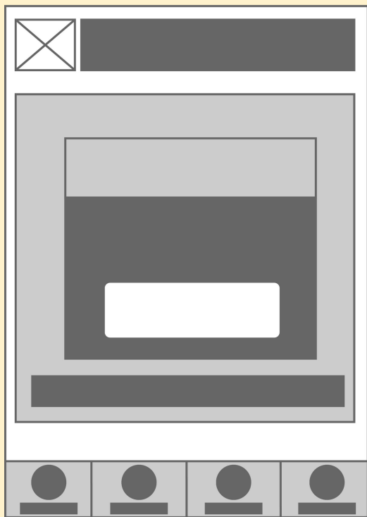
設定頁1
