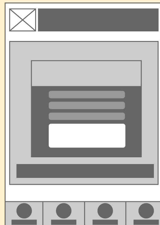
設定頁步驟6
