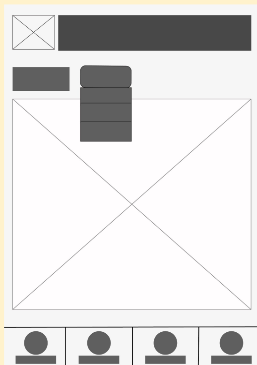
圖表分析
