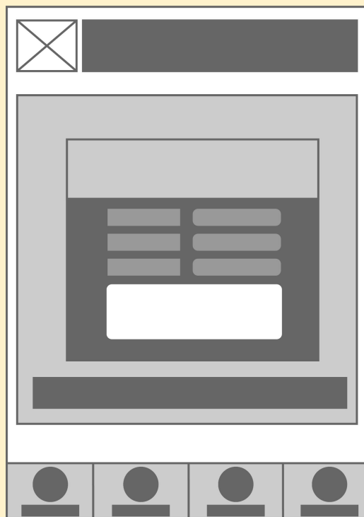
設定頁步驟5
