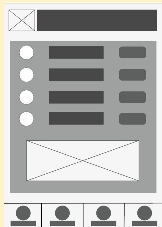
兌換中心
