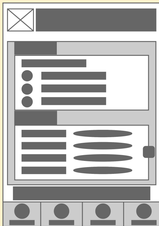
首頁1
