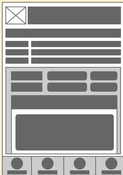
記帳頁
