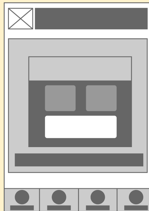
設定頁步驟3
