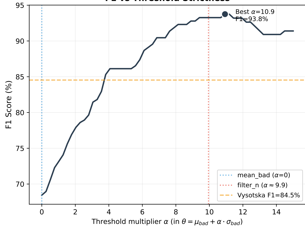
F1 vs Threshold Strictness
