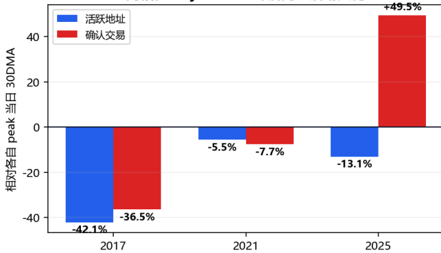
同相位 day +296：峰后高频活动变化
