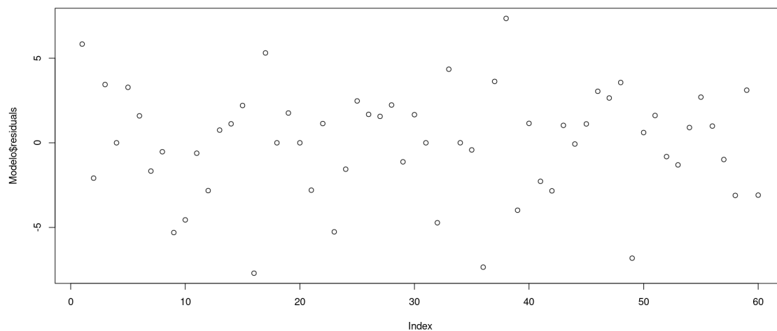
Figura 2: Gráfico de dispersión de los residuos del modelo factorial. Se observa la distribución de los residuos respecto a su índice, útil para verificar supuestos como homocedasticidad e independencia.
