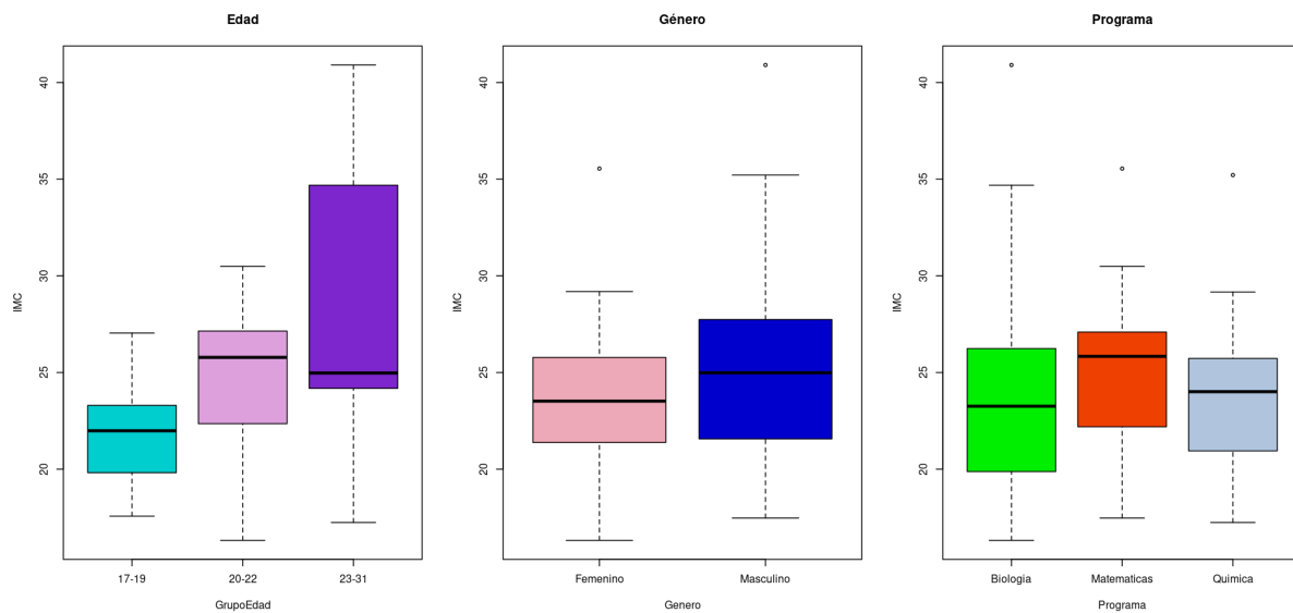
Figura 3: Boxplots del IMC según grupo de edad, género y programa académico. Este gráfico permite comparar visualmente la distribución y variabilidad del índice de masa corporal entre los distintos niveles de cada factor.
