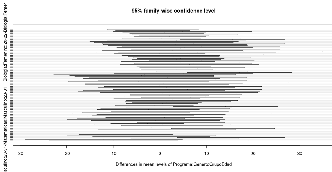
Figura 6: Comparaciones múltiples con intervalos de confianza del 95 % para la interacción Programa \times Género \times GrupoEdad.
