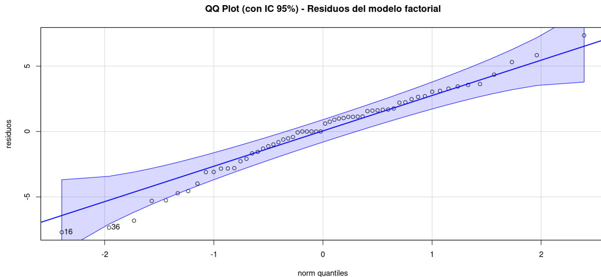
Figura 1: QQ Plot (con IC 95 %) de los residuos del modelo factorial. La línea azul representa la distribución normal teórica. Los puntos deben seguir esta línea si los residuos se distribuyen normalmente.
