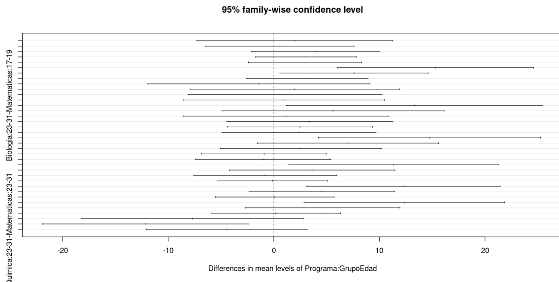
Figura 5: Intervalos de confianza del 95 % para las diferencias en los niveles medios de IMC según la interacción Programa \times GrupoEdad. .
