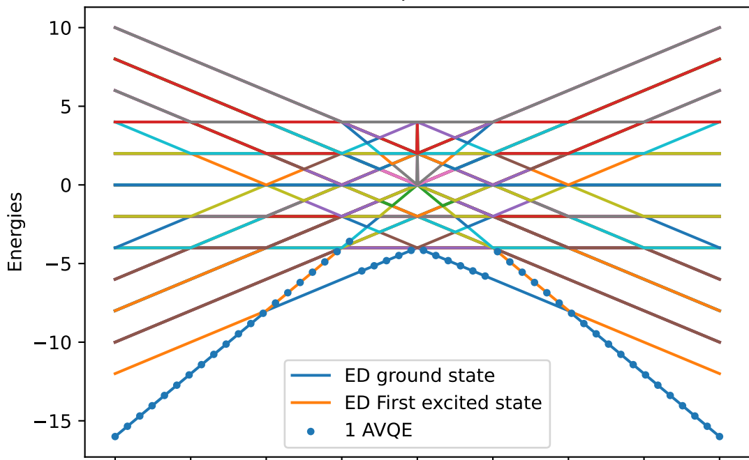
Adapt VQE
