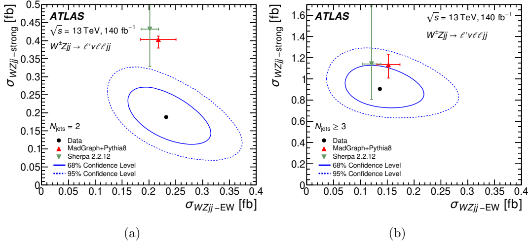
Figura 6: Sezioni d'urto misurate \sigma_{EW} e \sigma_{strong} per le categorie (a) N_{jet} = 2 e (b) N_{jet} \geq 3 , confrontate con le previsioni di MGPY8 e SHERPA 2.2.12. I contorni continui e tratteggiati corrispondono al 68% e 95% CL.
