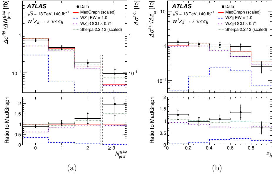
Figura 10: Sezione d'urto differenziale inclusiva di W^\pm Z jj misurata nello spazio delle fasi fiduciale del VBS in funzione di: (a) N_{\text{jet}}^{\text{gap}} (molteplicità esclusiva di jet con p_T > 25 \text{ GeV} nel gap di pseudorapidità tra i due jet di tagging ) e (b) \zeta_{j3} (variabile di Zeppenfeld per il terzo jet). Le definizioni delle barre di errore, delle linee e dei pannelli inferiori seguono la convenzione di Figura 8.
