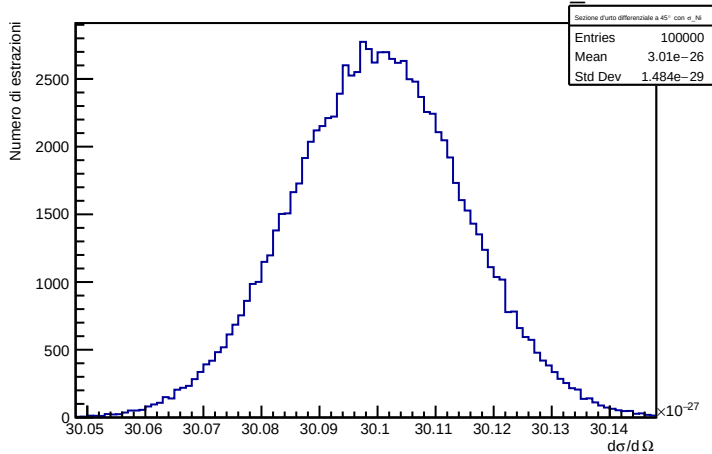
Sezione d'urto differenziale a 45° con \sigma_{\text{Ni}}
