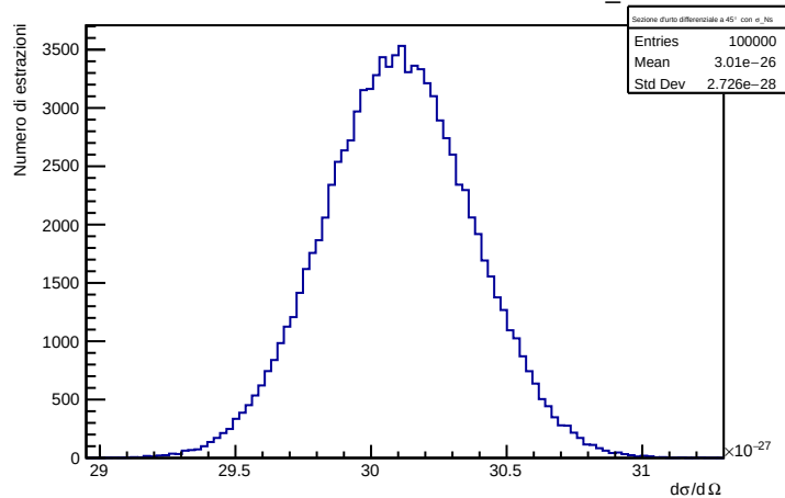
Sezione d'urto differenziale a 45° con \sigma_{\text{Ns}}
