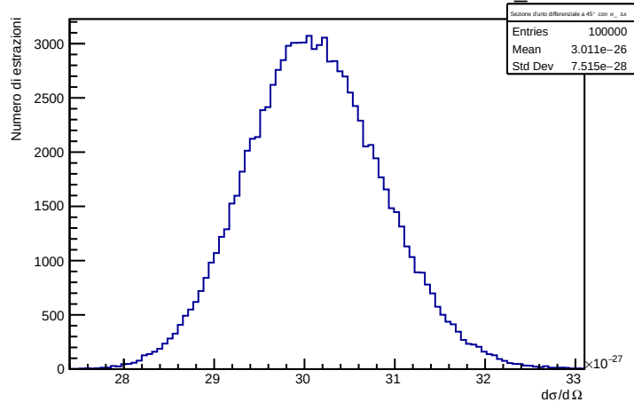
Sezione d'urto differenziale a 45° con \sigma_{\text{x}}
