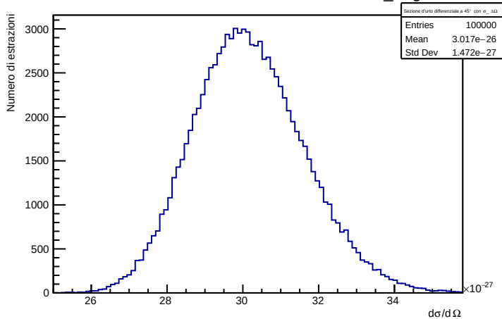
Sezione d'urto differenziale a 45° con \sigma_{\text{ang}}
