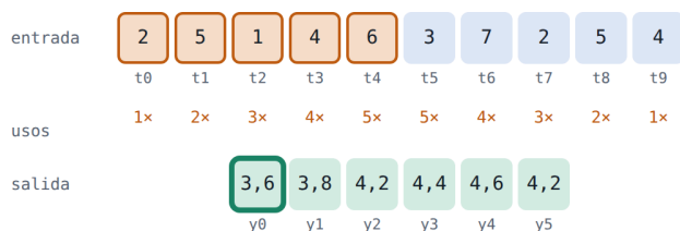
Figura 8. La misma señal sin padding. La salida se acorta 4 pasos, y la fila de usos muestra que los bordes se miran menos veces que el centro.
