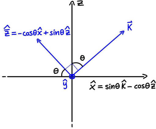
FIG. 5.2: cambio di sistema di riferimento (\hat{x}, \hat{y}, \hat{z}) \rightarrow (\hat{k}, \hat{y}, \hat{\bar{z}})
