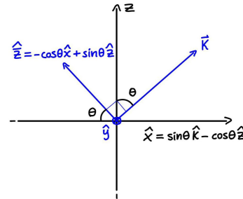
FIG. 5.1: cambio di sistema di riferimento (\hat{x}, \hat{y}, \hat{z}) \rightarrow (\hat{k}, \hat{y}, \hat{z})
