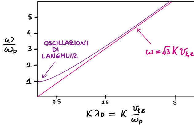
FIG. 2.1: Rappresentazione approssimativa della dispersione \frac{\omega}{\omega_p} = (1 + \gamma k^2 \lambda_D^2) . Non vi sono onde di Langmuir per \omega < \omega_p .
