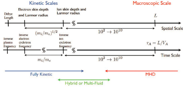
FIG. 2.1: lunghezze e tempi caratteristici, fonte: NationalAcademies.org
