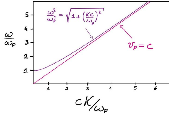
FIG. 2.2: Relazione di dispersione di onda e.m. trasversa ( \vec{k} \parallel \vec{E} )
