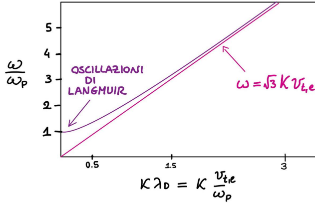
FIG. 2.1: Non vi sono onde di Langmuir per \omega < \omega_p .
