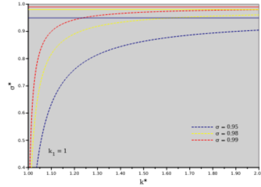
FIG. 13.1: convergenza di \sigma^* a \sigma .
