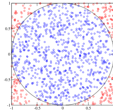
FIG. 1.7: Integrale Monte Carlo dell'area di un cerchio
