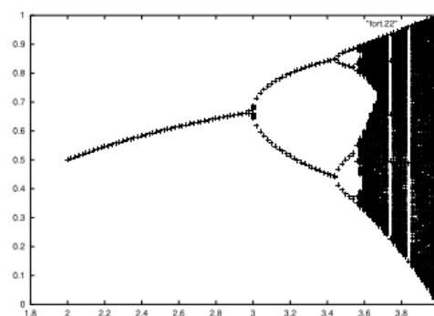
FIG. 1.2: La curva logistica, sembra di essere tornati a lezione da Paolini, wow
