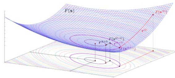
FIG. 11.3: Visualizzazione della discesa
