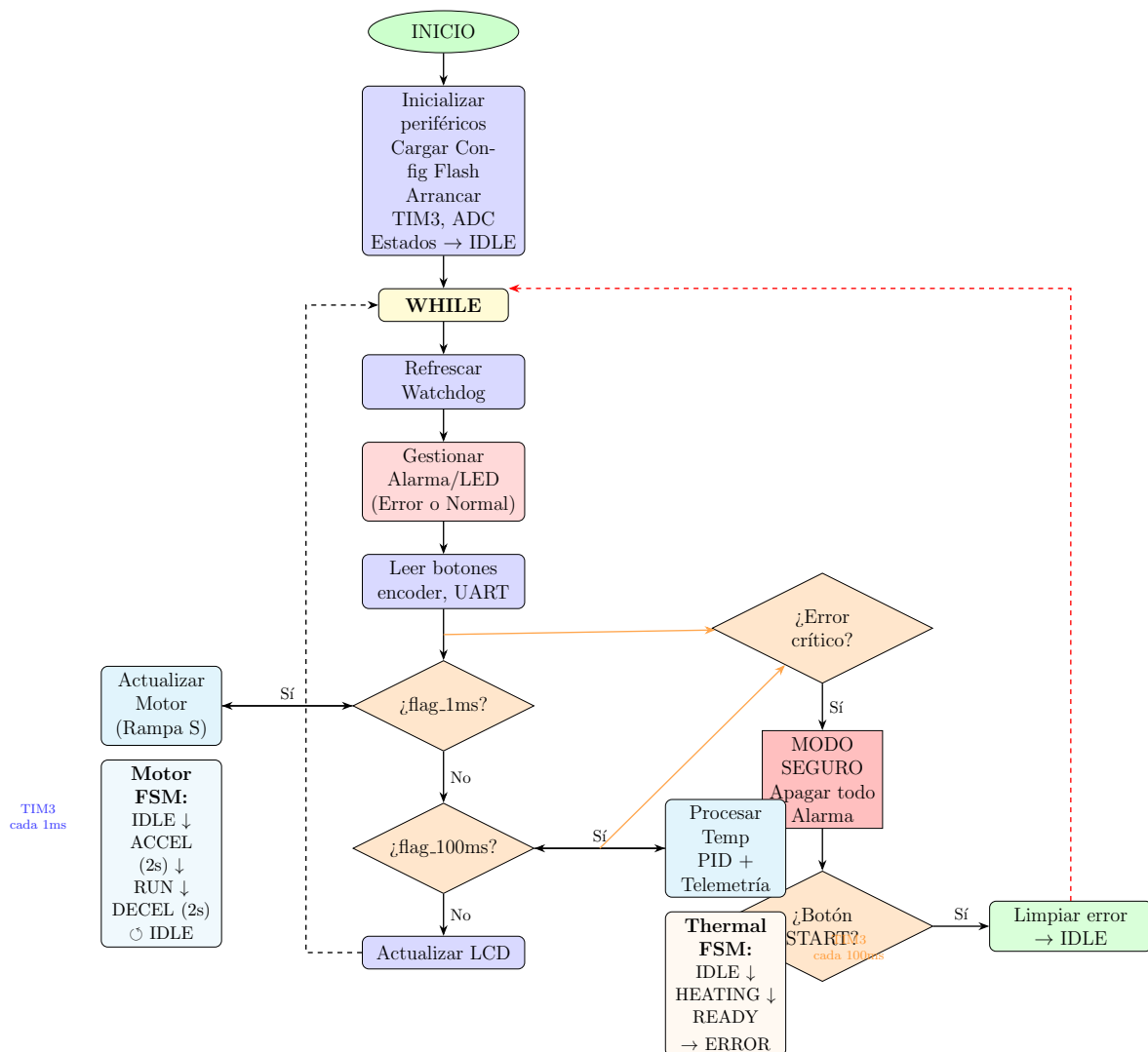
Figura 4: Diagrama de flujo del bucle principal y coordinación de máquinas de estado.
