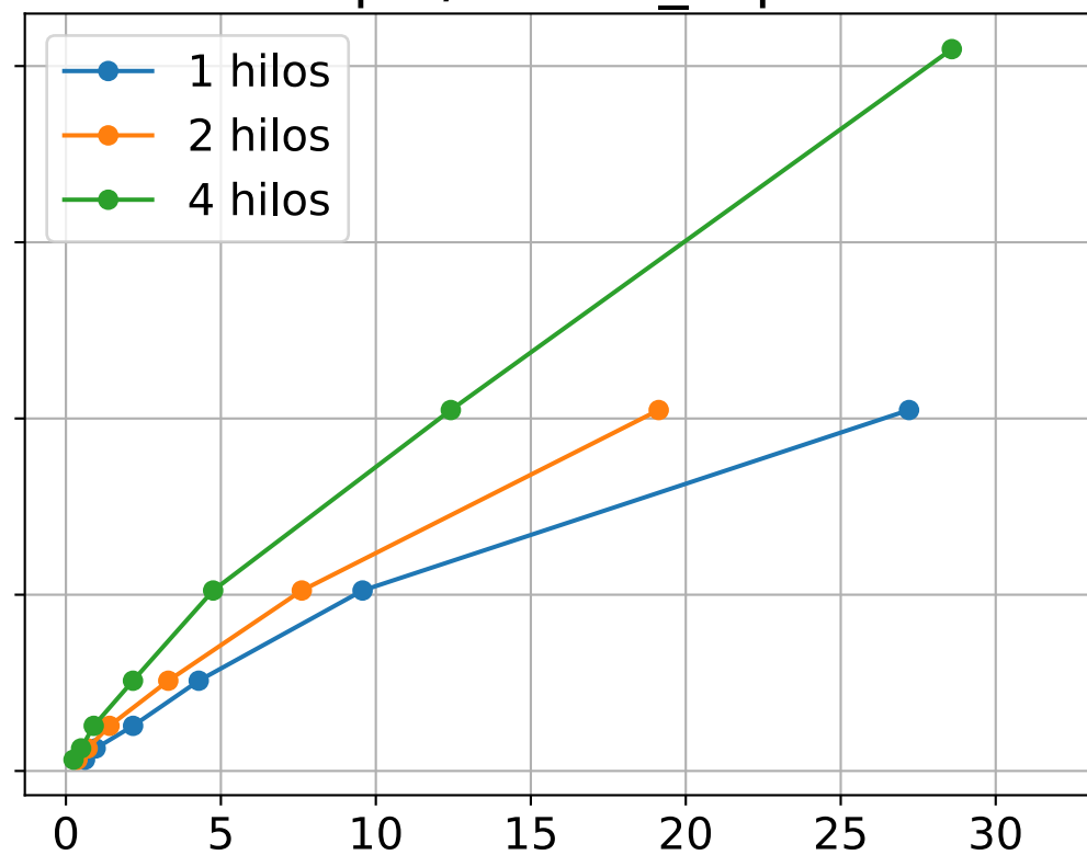
rpi4/results_sap
