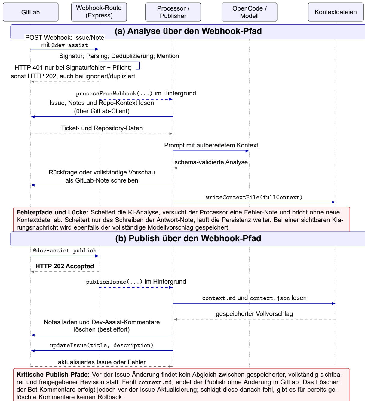
Abbildung 4.2.: Sequenz der Analyse- und Publish-Verarbeitung über den GitLab-Webhook. Die Route bestätigt angenommene Ereignisse früh mit HTTP 202 und führt Process beziehungsweise Publish anschließend ohne Rückkanal zum Aufrufer aus. Rote Hinweise kennzeichnen implementierte Fehlerpfade und die fehlende Kopplung zwischen sichtbarer Vorschau, gespeichertem Kontext und Freigabe. Eigene Darstellung auf Grundlage des untersuchten Quellcodes, Stand 31.07.2026.
