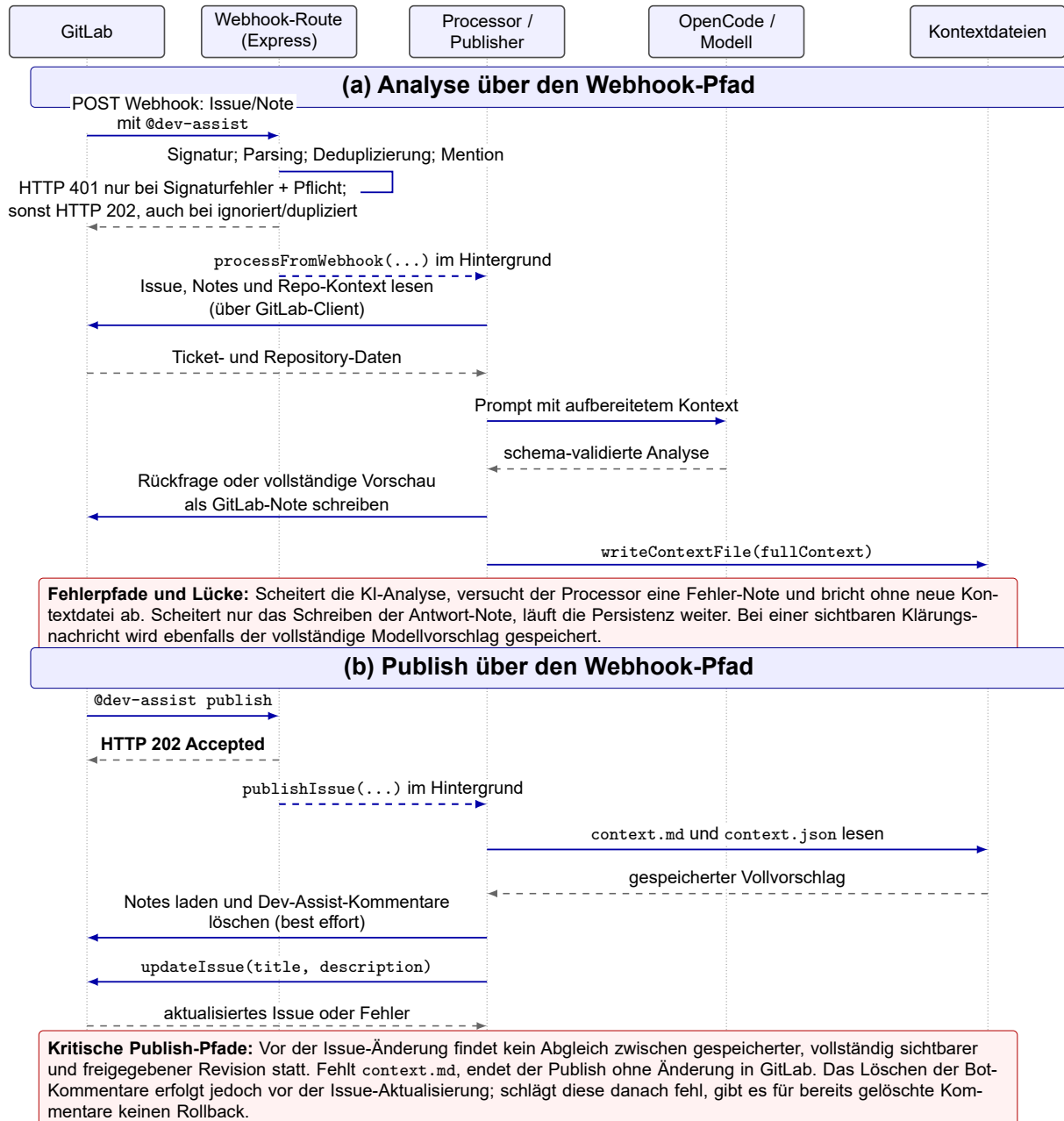
Abbildung 4.2.: Sequenz der Analyse- und Publish-Verarbeitung über den GitLab-Webhook. Die Route bestätigt angenommene Ereignisse früh mit HTTP 202 und führt Prozess beziehungsweise Publish anschließend ohne Rückkanal zum Aufrufer aus. Rote Hinweise kennzeichnen implementierte Fehlerpfade und die fehlende Kopplung zwischen sichtbarer Vorschau, gespeichertem Kontext und Freigabe. Eigene Darstellung auf Grundlage des untersuchten Quellcodes, Stand 31.07.2026.
